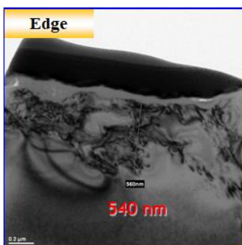
Resin #325, edge: 540 nm.
