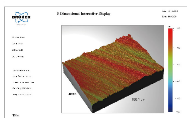
Edge surface: Ra 1.17 nm.
