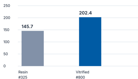
Die strength after Z1 [MPa]
