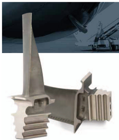
Turbinenschaufeln und profilierte Schaufelfüße
