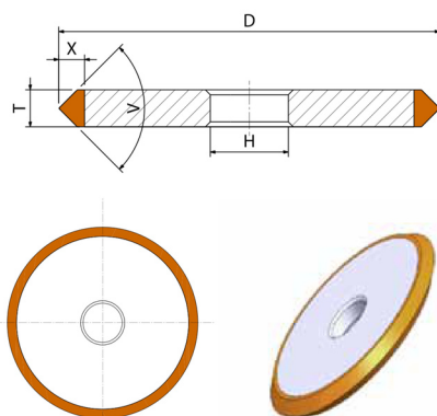
1E1: Querschnitt, Maßkennungen und Werkzeugdarstellung
