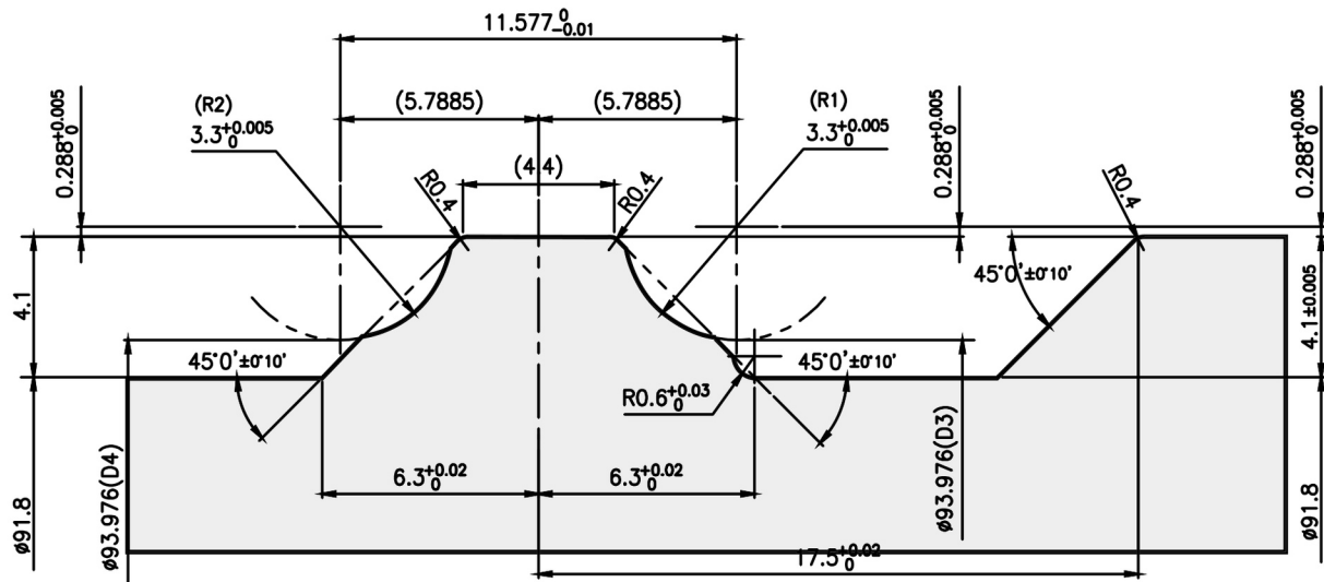
Schienenprofil: Maße, Radien und Winkeltoleranzen
