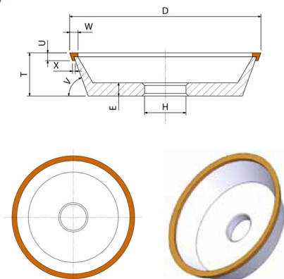
11Y9: Querschnitt, Maßkennungen und Werkzeugdarstellung
