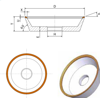
12V4: Querschnitt, Maßkennungen und Werkzeugdarstellung
