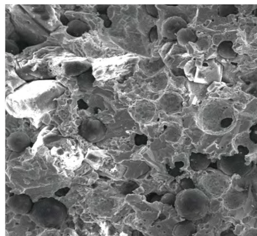
Poröse Hybridbindung: Gefügaufnahme 2
