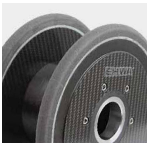
Keramisch gebundene Schleifscheiben mit CFK-Grundkörper
