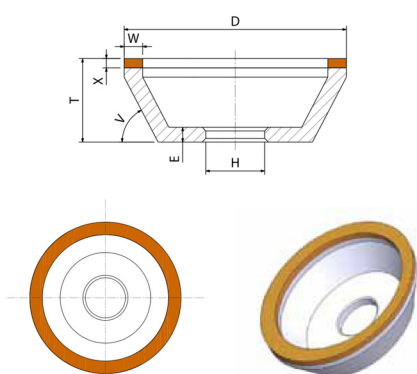
11A2: Querschnitt, Maßkennungen und Werkzeugdarstellung
