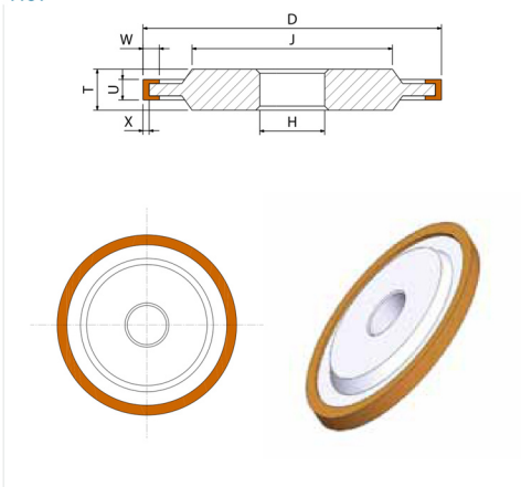
14U1: Querschnitt, Maßkennungen und Werkzeugdarstellung
