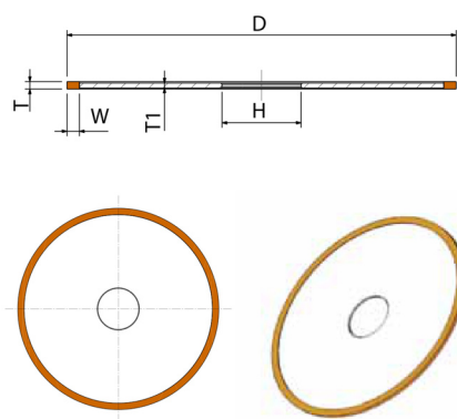
1A1R: Querschnitt, Maßkennungen und Werkzeugdarstellung
