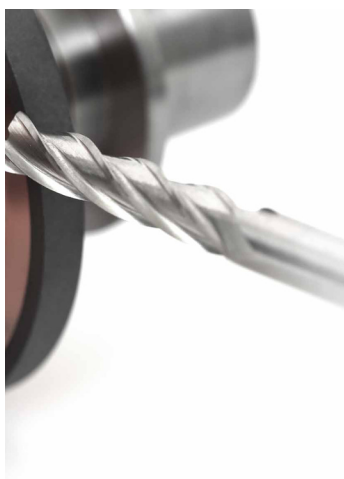
Superabrasive Scheibe bei der Werkzeugbearbeitung
