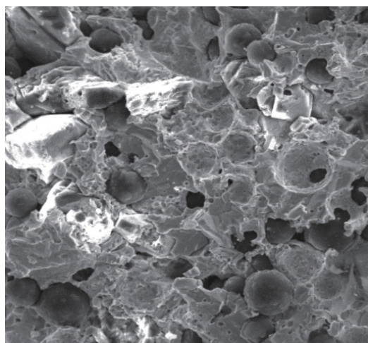
Poröse Hybridbindung: Gefügeaufnahme 2
