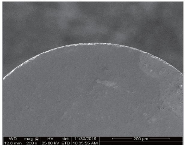
Kantenaufnahme im Hybridbindungs-Anwendungsbeispiel
