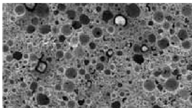
CBN-Honstein: grobe Porenstruktur
