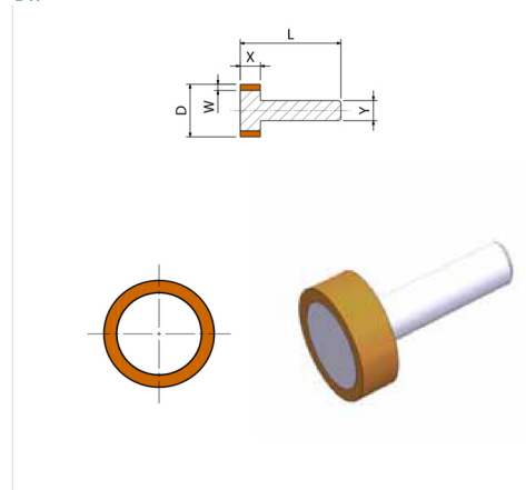
DW: Querschnitt, Maßkennungen und Werkzeugdarstellung
