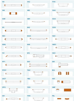
Werkzeugquerschnitte
