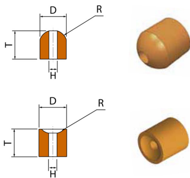
BUL: Querschnitt, Maßkennungen und Werkzeugdarstellung
