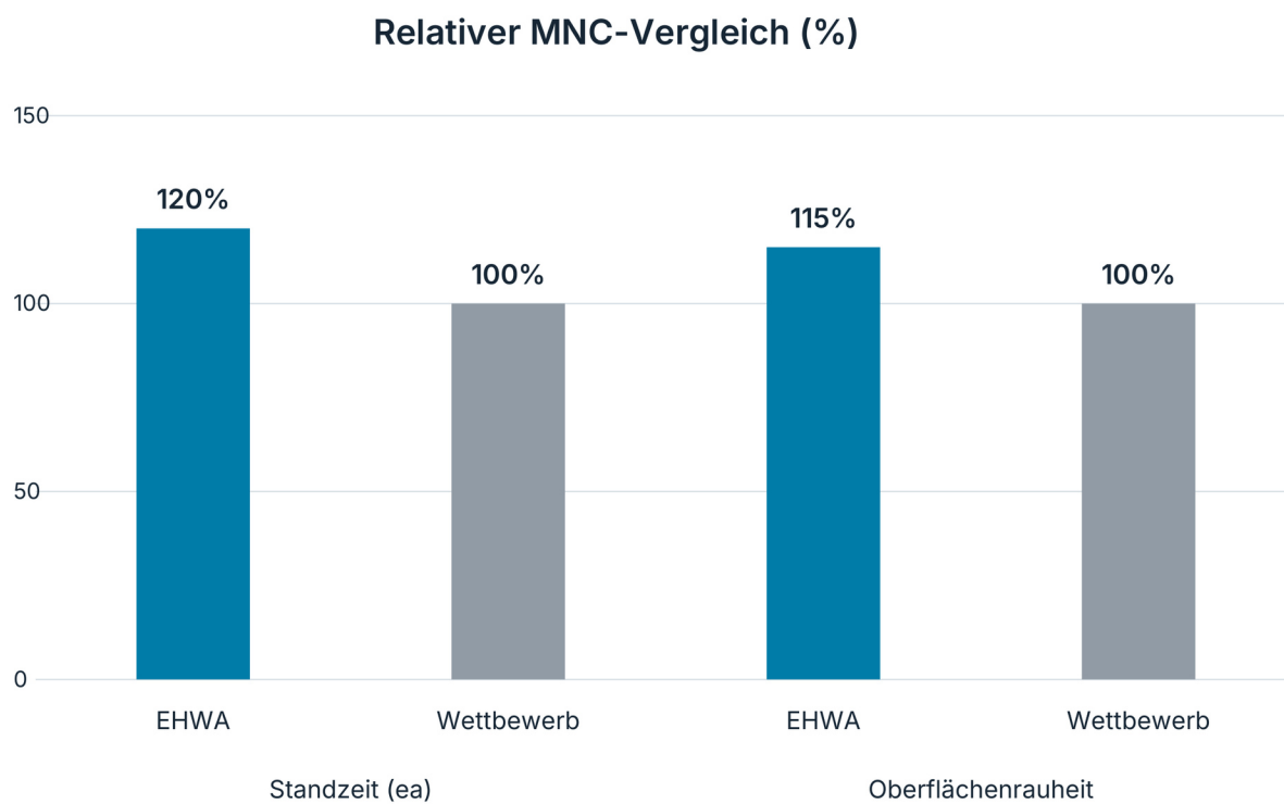
Relativer MNC-Vergleich: Standzeit und Quellenindex zur Oberfläche
