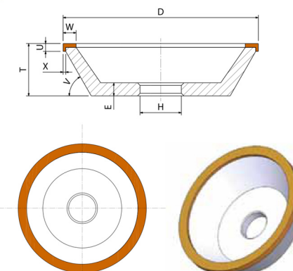
11C9: Querschnitt, Maßkennungen und Werkzeugdarstellung
