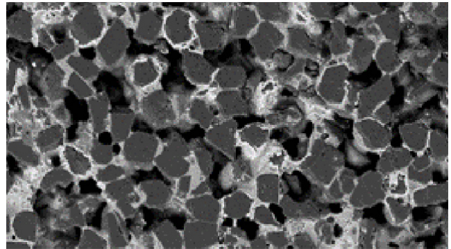
CBN-Struktur für die Käfigfenster-Bearbeitung.
