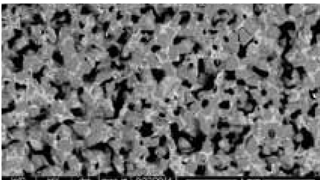
Porenstruktur der keramisch gebundenen Scheibe für den Außenring.
