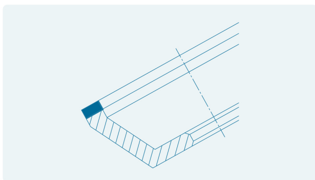
Werkzeugquerschnitte: Geometrie als Grundlage der Spezifikation
