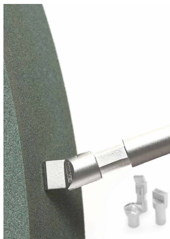
Stationäres Diamantabrichten: Abrichter und Schleifscheibe
