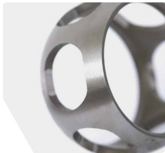
Rotierender Abrichter und Gleichlaufgelenk-Käfig.
