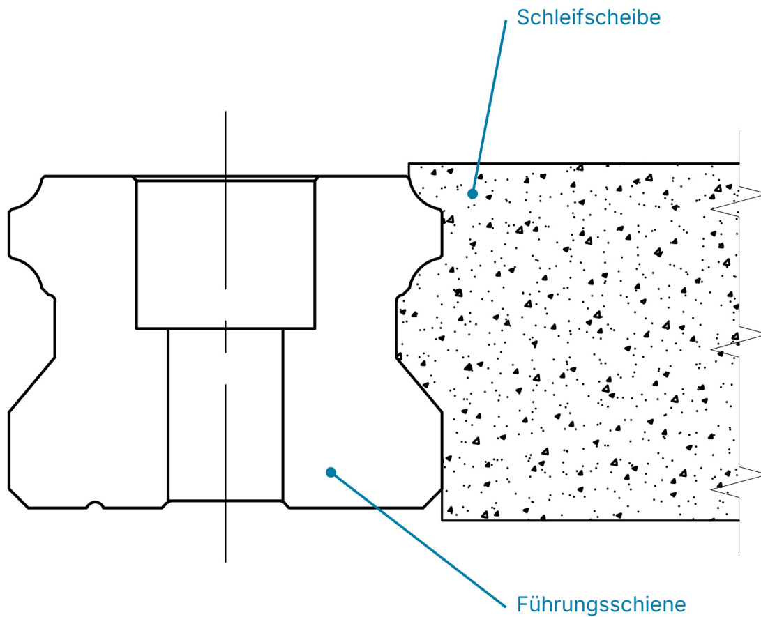
Schleifscheibe und Führungsschiene im Profilkontakt
