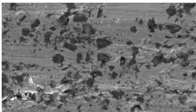
Gefüge einer Hybridbindung
