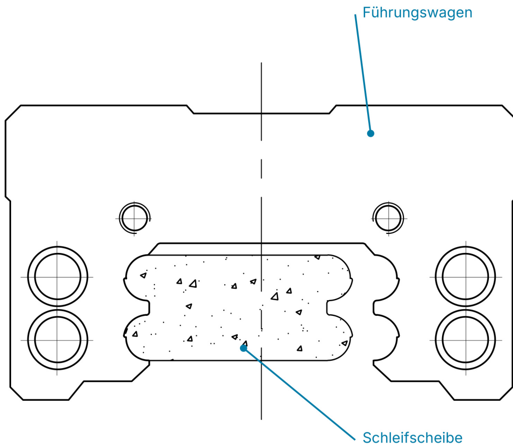
Schleifscheibe und Führungswagen im Profilkontakt
