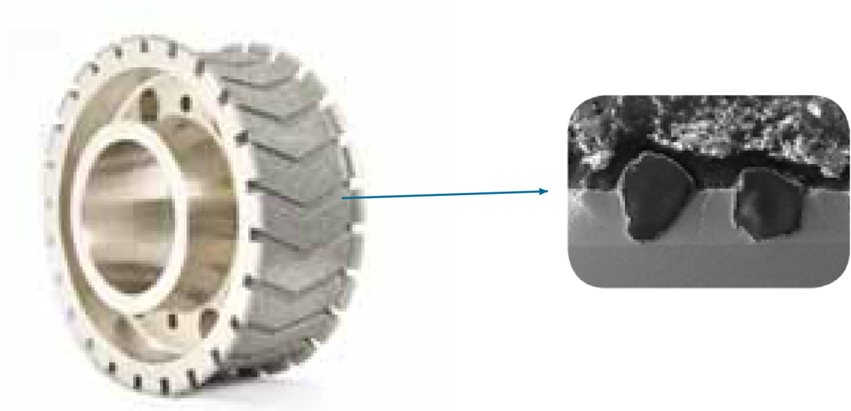
Galvanisch belegt: Schleifscheibe und Schleifbelag im Detail.
