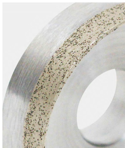
Diamantbelag eines Topf-Abrichters
