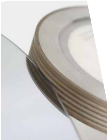
Metallgebundene Kantenschleifscheibe für Außenspiegel
