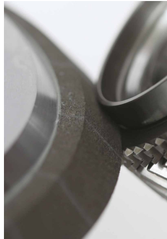
Profilierte Schleifwerkzeuge und Belagstruktur
