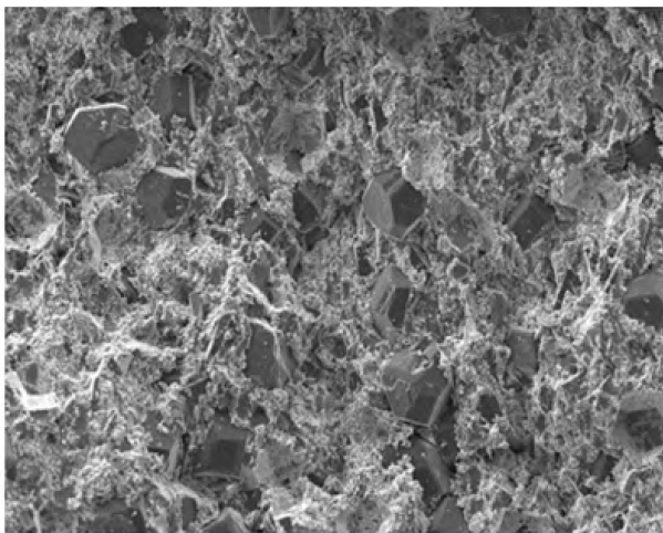
Gefüge der MNC-Bindung
