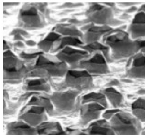
Oberflächenstruktur einer Linsenschleifscheibe
