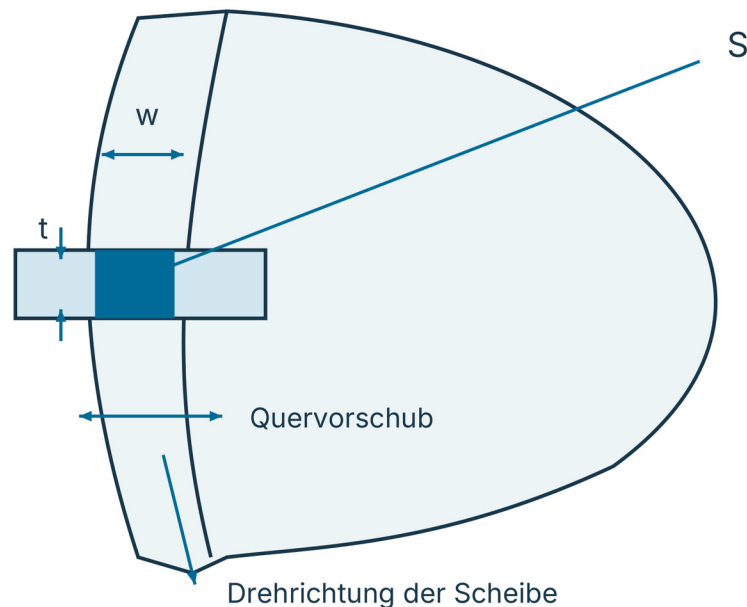
Kontaktfläche S, Belagbreite w und Kontaktlänge t
