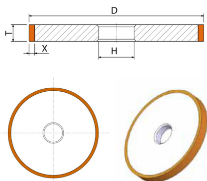
1A1: Querschnitt, Maßkennungen und Werkzeugdarstellung
