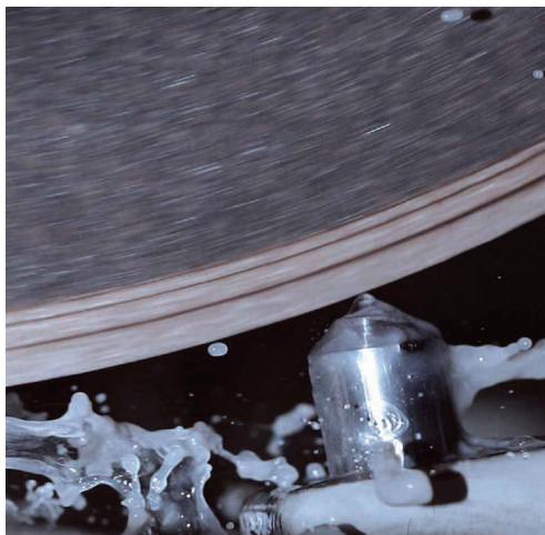
Stationäres Diamantabrichten mit Kühlschmierstoff
