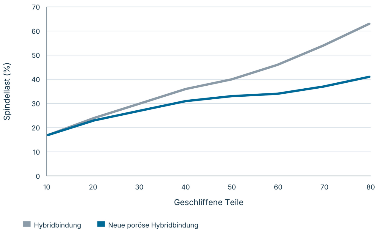
Spindellast über der Zahl geschliffener Teile: Hybrid und neue poröse Hybridbindung
