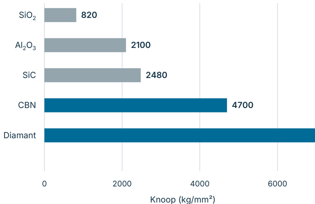
Härtevergleich der Schleifstoffe: Knoop-Skala
