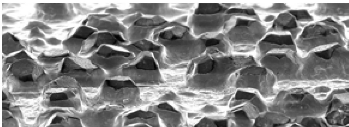
Strukturaufnahme der BSL-Schleifscheibe mit Schlitzten.
