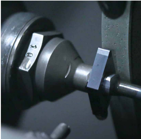
Umfangsschleifen einer Schneidplatte
