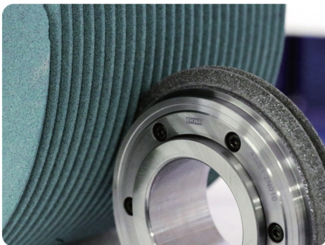
Abrichtrolle im Zahnrad-Schleifprozess
