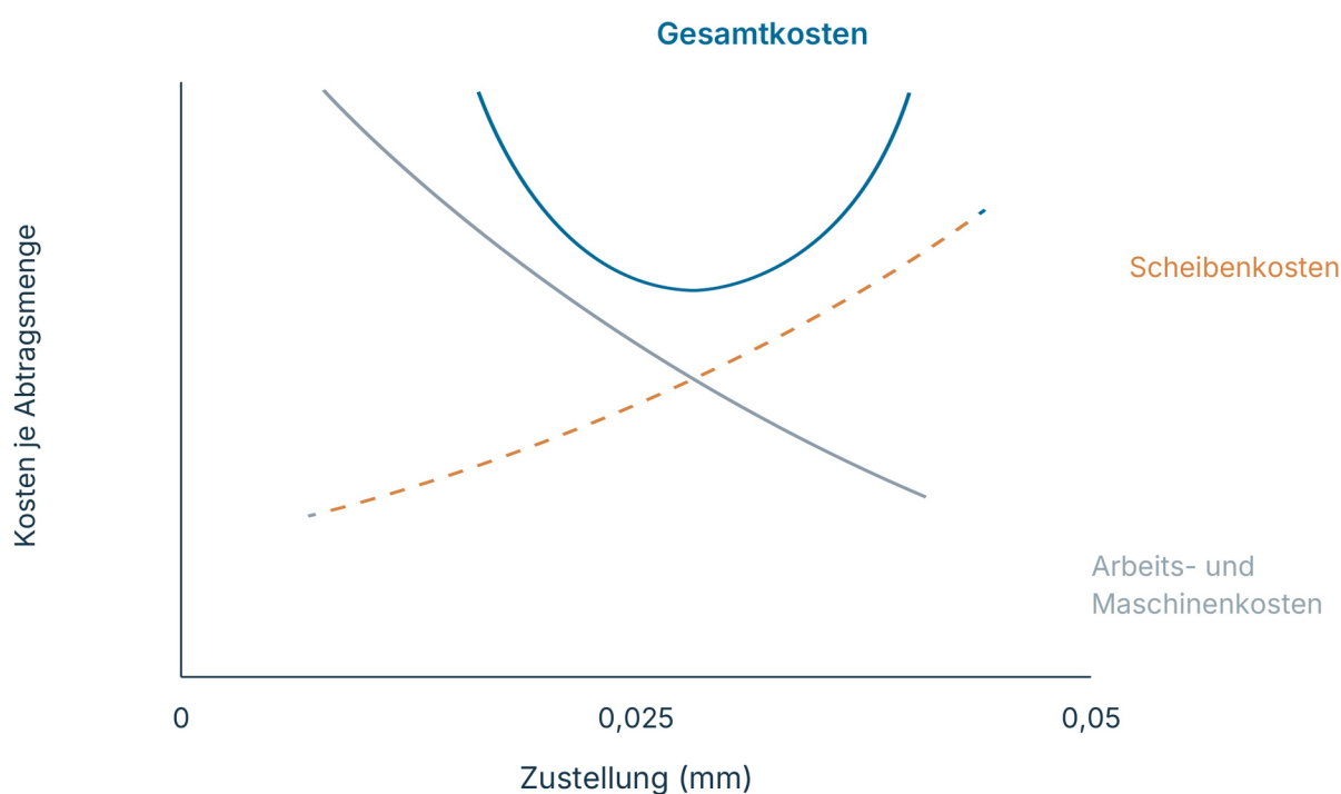
Schematische Bearbeitungskosten über der Zustellung
