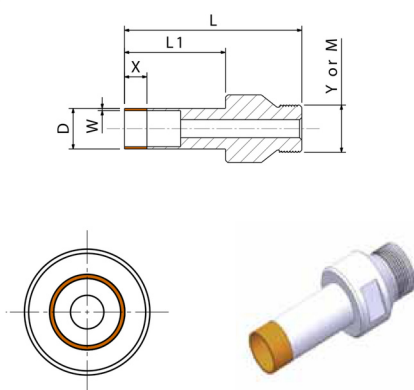
6F2: Querschnitt, Maßkennungen und Werkzeugdarstellung
