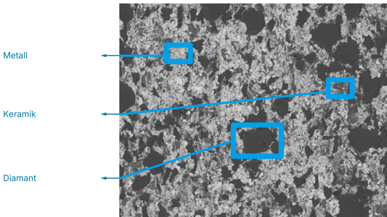
MNC-Gefüge: Metall, keramische Phase und Diamant
