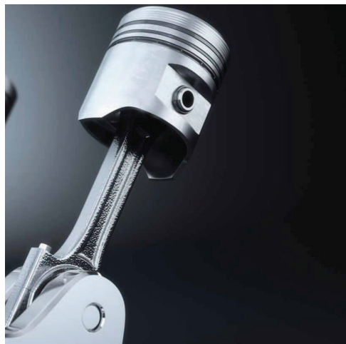
Kolben und Pleuel als Motor-Anwendungsbeispiel.
