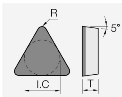
TBGN (PCBN): Schneidplattenmaßzeichnung mit den zugehörigen Geometriezeichen.
