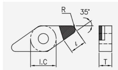
VNGA (PCD / CVD): Schneidplattenmaßzeichnung mit den zugehörigen Geometriezeichen.
