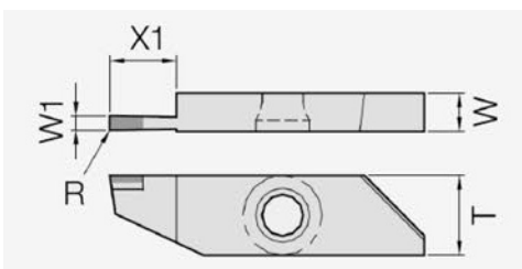
EMG-Ausführung: isoliertes Maßschema.
