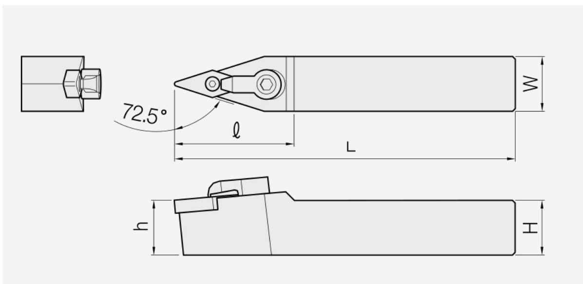
MVWNN: Haltermaßzeichnung; Artikelmaße und Ersatzteile stehen in den zugehörigen Tabellen.
