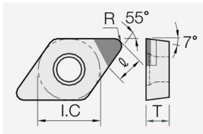
DCGW (PCD / CVD): Schneidplattenmaßzeichnung mit den zugehörigen Geometriezeichen.
