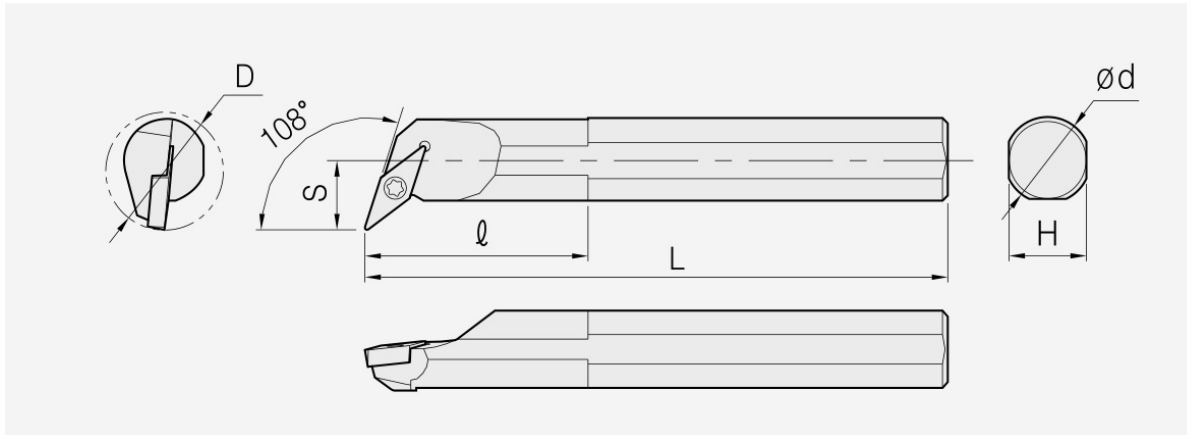
SVQC: Haltermaßzeichnung; Artikelmaße und Ersatzteile stehen in den zugehörigen Tabellen.
