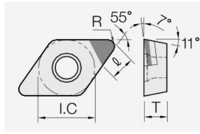
DPGT (PCD / CVD): Schneidplattenmaßzeichnung mit den zugehörigen Geometriezeichen.
