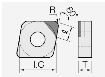
CNGA (PCBN): Schneidplattenmaßzeichnung mit den zugehörigen Geometriezeichen.
