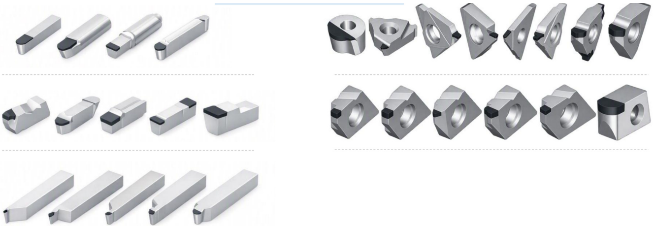
Übersicht kundenspezifischer Werkzeugformen.
