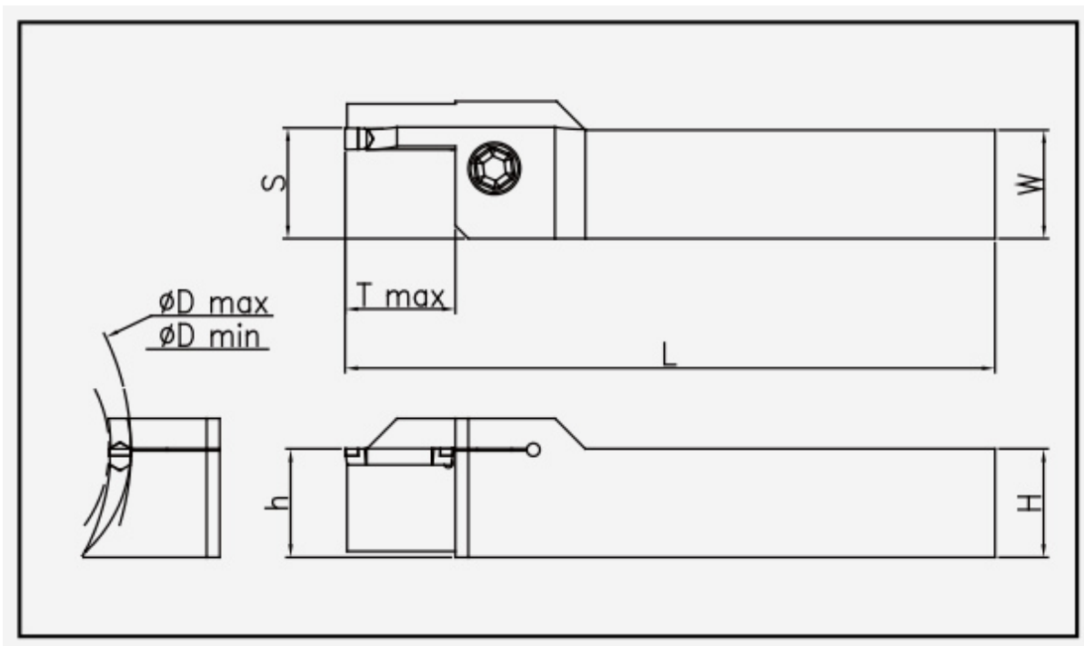
ESFH: Haltermaßzeichnung; Artikelmaße und Ersatzteile stehen in den zugehörigen Tabellen.
