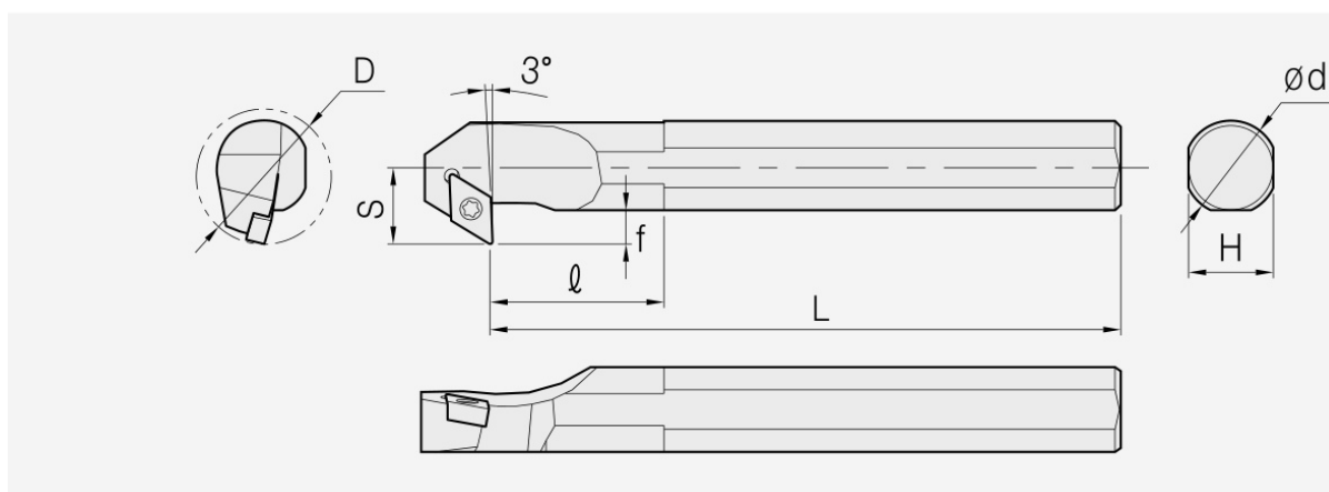
SDZC: Haltermaßzeichnung; Artikelmaße und Ersatzteile stehen in den zugehörigen Tabellen.
