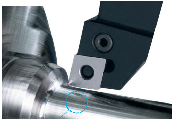
Illustrative Bearbeitungsansicht mit Wiper.
