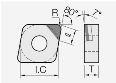
CNGX (PCD / CVD): Schneidplattenmaßzeichnung mit den zugehörigen Geometriezeichen.
