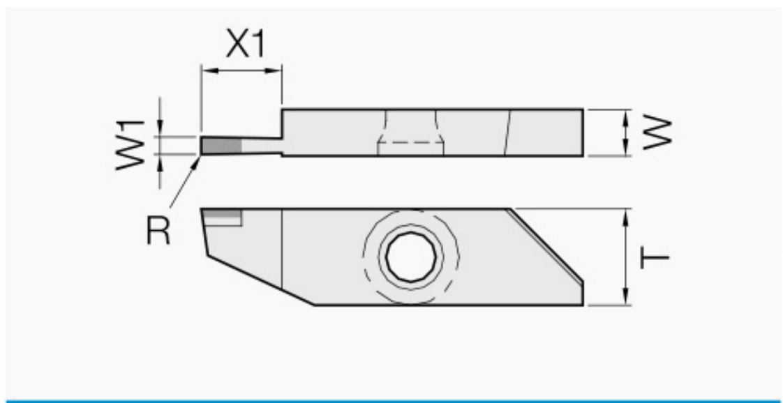
Schneidplatte: isoliertes Maßbild mit unveränderten Geometriezeichen.
