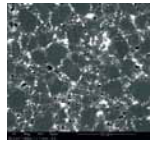
PKD: Korngröße, Diamantanteil und Sortenauswahl: Gefügeaufnahme mit dem dargestellten Maßstab.
