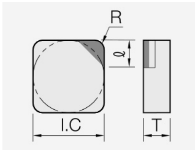
SNGN (PCBN): Schneidplattenmaßzeichnung mit den zugehörigen Geometriezeichen.
