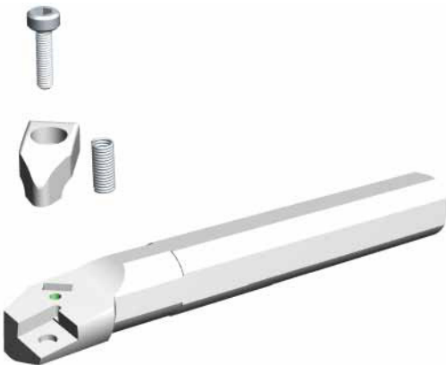
Innenhalter: Doppel- und Mehrfachspannung: Werkzeugansicht.
