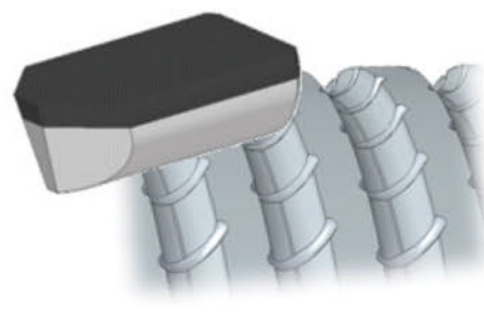
PKD-Sorten EP20, EP55 und EP59: Bauteil- und Bearbeitungsansicht.
