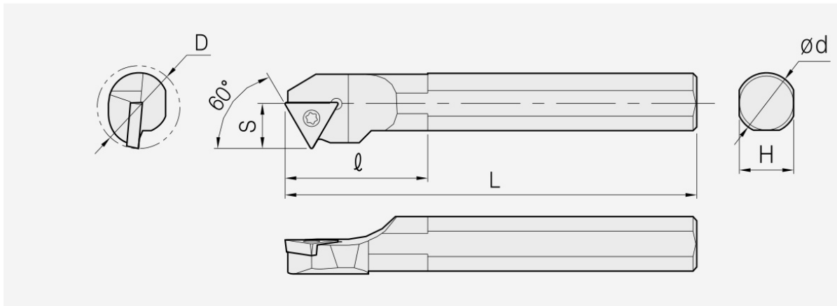
STWP: Haltermaßzeichnung; Artikelmaße und Ersatzteile stehen in den zugehörigen Tabellen.
