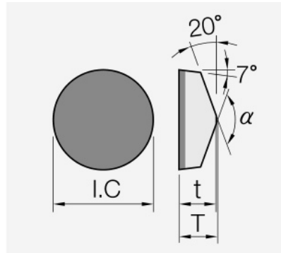
Schneidplatte: isoliertes Maßbild mit unveränderten Geometriezeichen.
