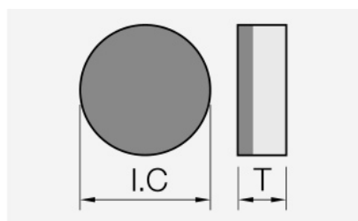
RNGN (PCD / CVD): Schneidplattenmaßzeichnung mit den zugehörigen Geometriezeichen.
