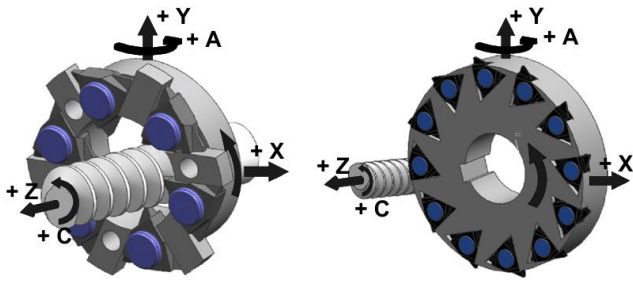
EB12-Wirbelwerkzeuge mit Achsendarstellung.
