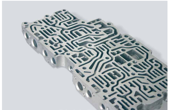
Ventilgehäuse aus Aluminiumlegierung: Bauteil- und Bearbeitungsansicht.
