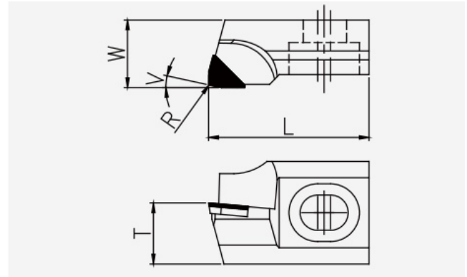
Schneidplatte: isoliertes Maßbild mit unveränderten Geometriezeichen.
