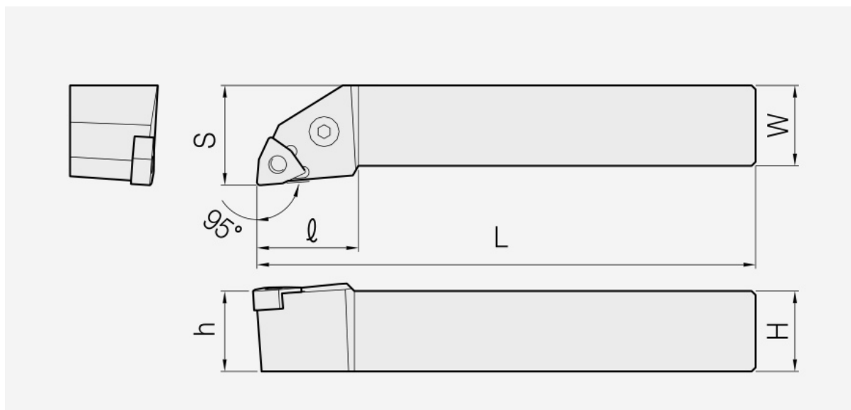
PWLN: Haltermaßzeichnung; Artikelmaße und Ersatzteile stehen in den zugehörigen Tabellen.
