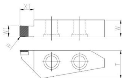
EMG3: bemaßte Werkzeugzeichnung.
