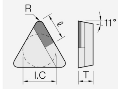
TPGN (L) (PCD / CVD): Schneidplattenmaßzeichnung mit den zugehörigen Geometriezeichen.
