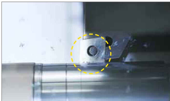
PCBN-Spanbrecher: SCM420-Anwendungsbeispiele: Bauteil- und Bearbeitungsansicht.
