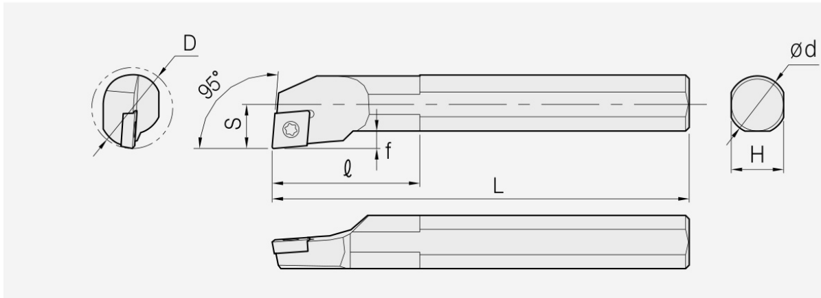
SCLC: Haltermaßzeichnung; Artikelmaße und Ersatzteile stehen in den zugehörigen Tabellen.
