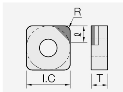
SNGA (PCBN): Schneidplattenmaßzeichnung mit den zugehörigen Geometriezeichen.
