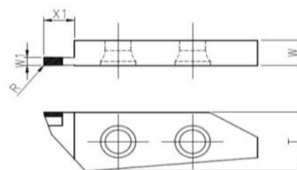
EMG2: bemaßte Werkzeugzeichnung.
