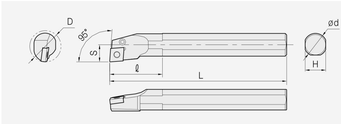
PCLN: Haltermaßzeichnung; Artikelmaße und Ersatzteile stehen in den zugehörigen Tabellen.
