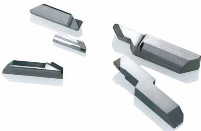
Ausdrehen: Stahl- und Hartmetallkörper: Werkzeugansicht.
