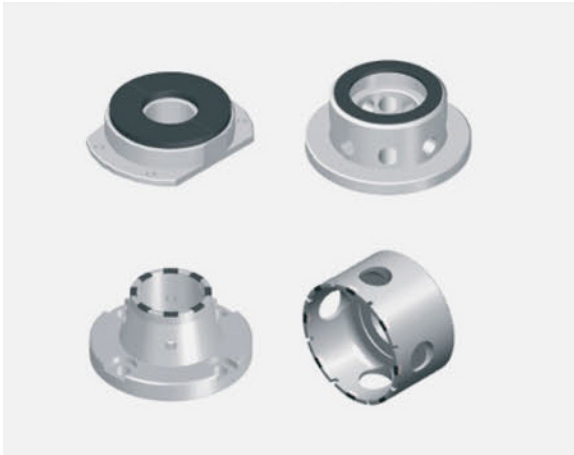
Verschleißteile für Schleif- und Messmaschinen: Werkzeugansicht.
