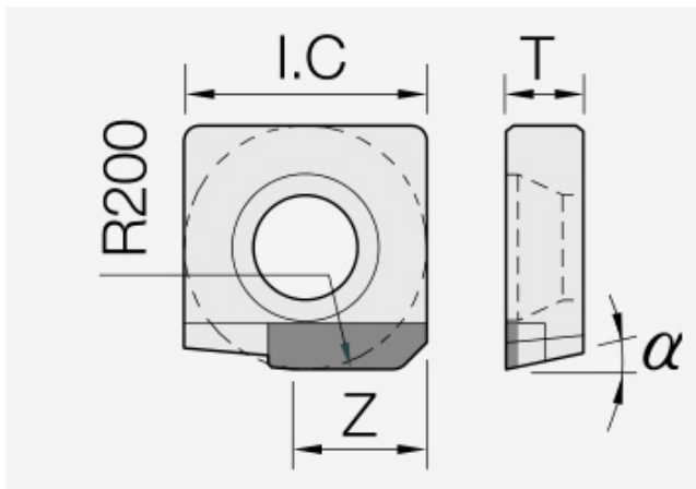
Schneidplatte: isoliertes Maßbild mit unveränderten Geometriezeichen.
