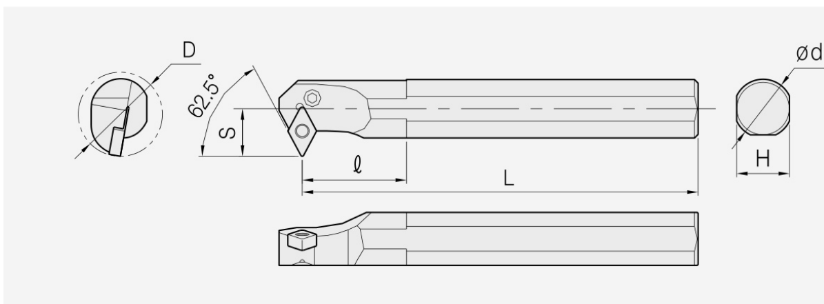
PDSN: Haltermaßzeichnung; Artikelmaße und Ersatzteile stehen in den zugehörigen Tabellen.
