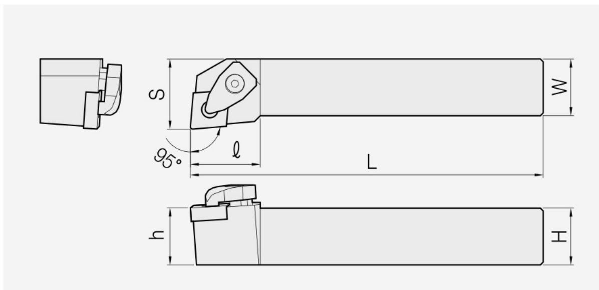
DCLN: Haltermaßzeichnung; Artikelmaße und Ersatzteile stehen in den zugehörigen Tabellen.
