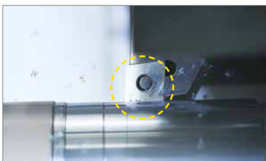
PCBN-Spanbrecher: SCM420-Anwendungsbeispiele: Bauteil- und Bearbeitungsansicht.
