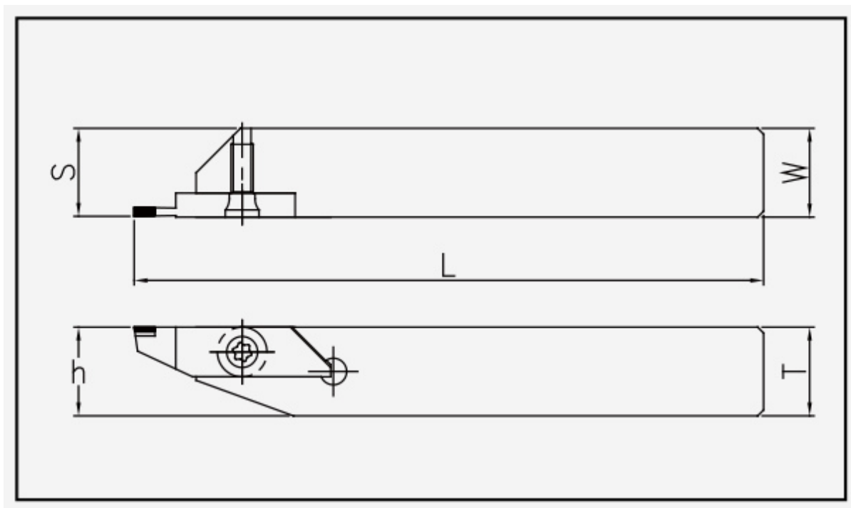
EMEH: Haltermaßzeichnung; Artikelmaße und Ersatzteile stehen in den zugehörigen Tabellen.
