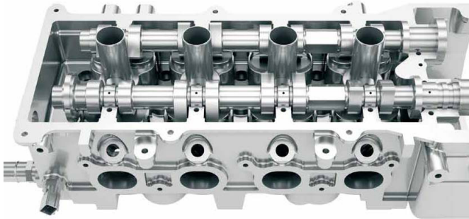
Rotierende Werkzeuge: Bauteil- und Bearbeitungsansicht.
