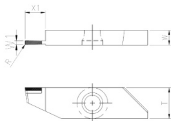
EMG: bemaßte Werkzeugzeichnung.
