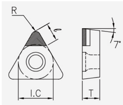
TCGW (PCBN): Schneidplattenmaßzeichnung mit den zugehörigen Geometriezeichen.
