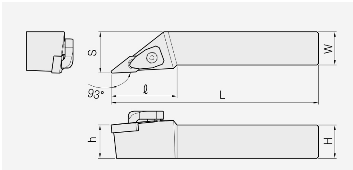
DVJN: Haltermaßzeichnung; Artikelmaße und Ersatzteile stehen in den zugehörigen Tabellen.
