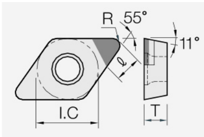
DPGW (PCD / CVD): Schneidplattenmaßzeichnung mit den zugehörigen Geometriezeichen.
