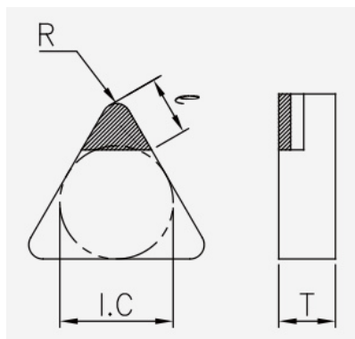
TNGN (PCBN): Schneidplattenmaßzeichnung mit den zugehörigen Geometriezeichen.
