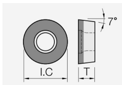
RCGW (PCD / CVD): Schneidplattenmaßzeichnung mit den zugehörigen Geometriezeichen.
