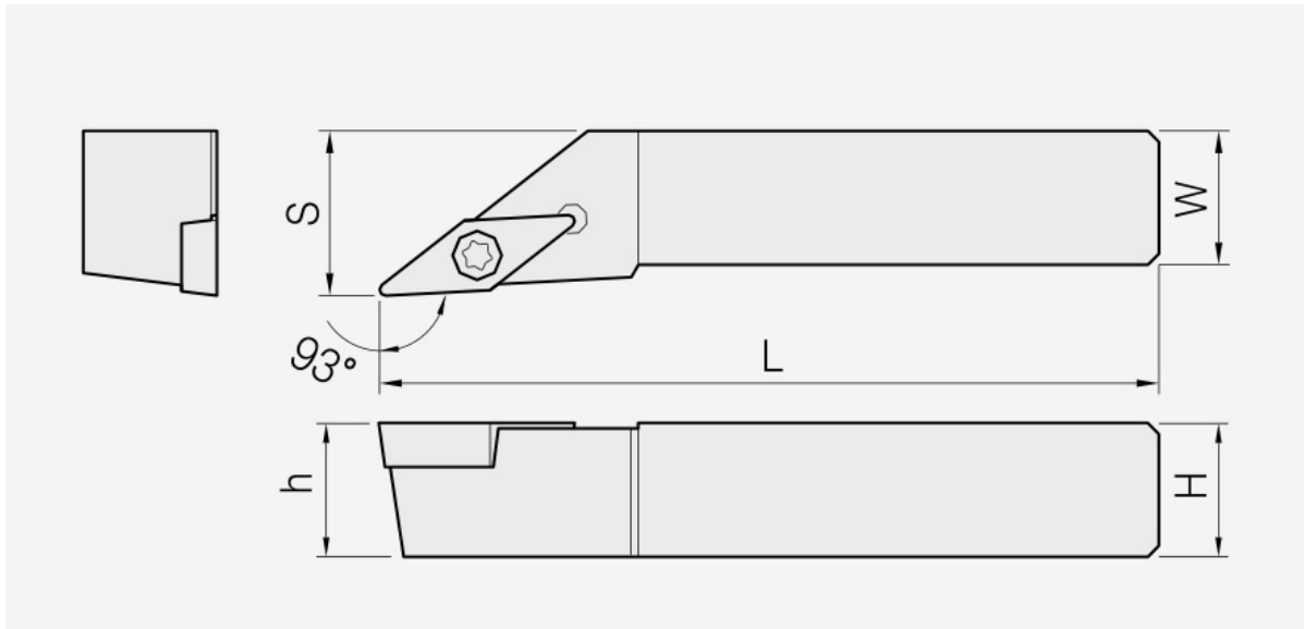
SVJB: Haltermaßzeichnung; Artikelmaße und Ersatzteile stehen in den zugehörigen Tabellen.
