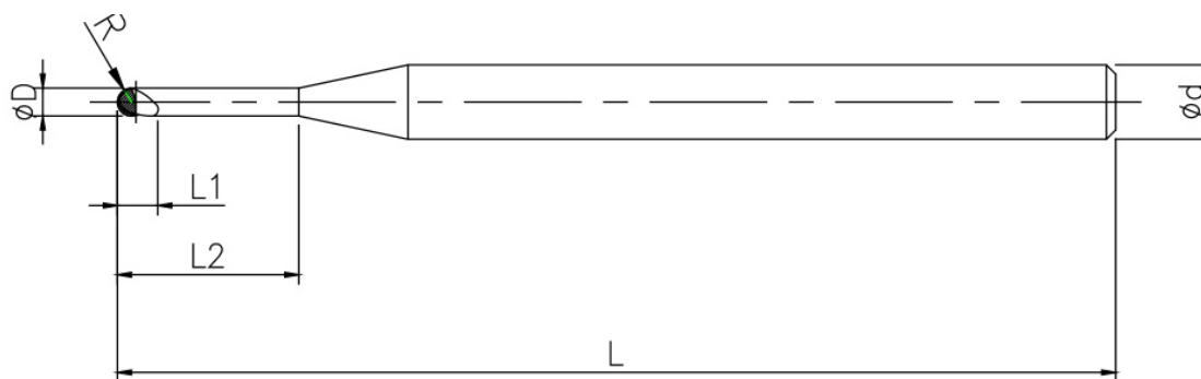
EBEB: PCBN-Kugelfräser: Werkzeugansicht.
