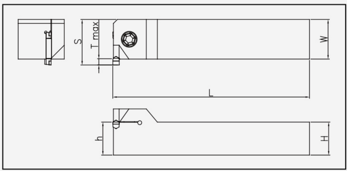
ESEV: Haltermaßzeichnung; Artikelmaße und Ersatzteile stehen in den zugehörigen Tabellen.
