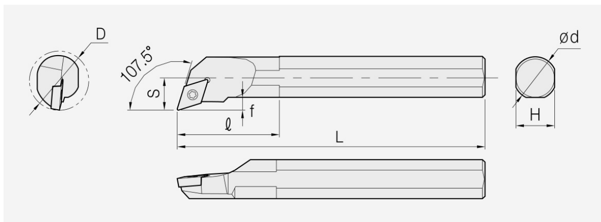
SDQC: Haltermaßzeichnung; Artikelmaße und Ersatzteile stehen in den zugehörigen Tabellen.
