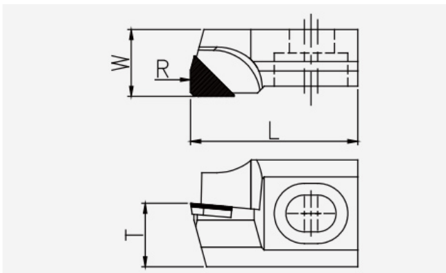
Schneidplatte: isoliertes Maßbild mit unveränderten Geometriezeichen.
