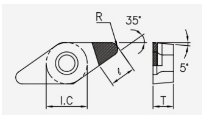
VBGW (PCD / CVD): Schneidplattenmaßzeichnung mit den zugehörigen Geometriezeichen.
