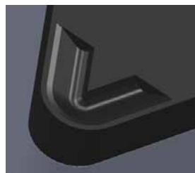
PKD-/CVD-Spanbrecher ER und EX: Werkzeugansicht.
