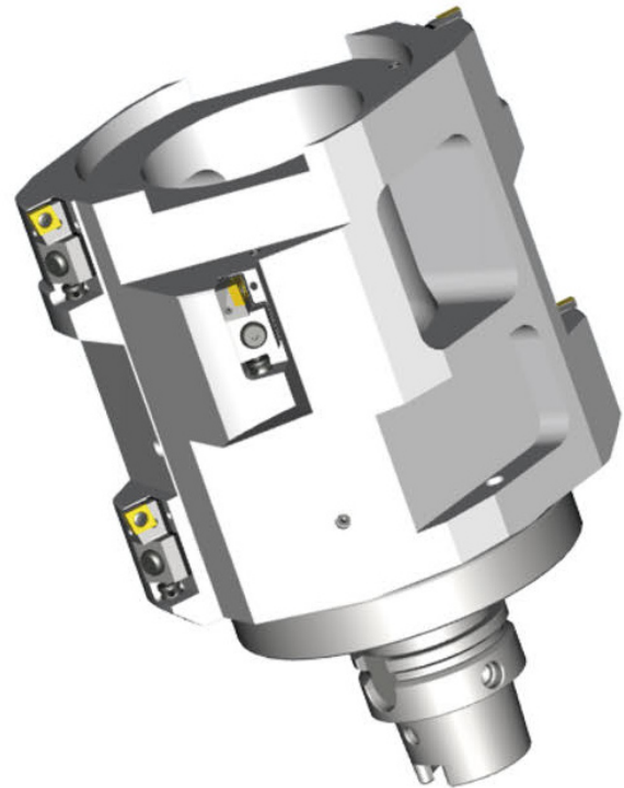
Spezial-Ausdrehwerkzeug für Motorgehäuse: Werkzeugansicht.
