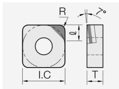
SNGX (PCD / CVD): Schneidplattenmaßzeichnung mit den zugehörigen Geometriezeichen.
