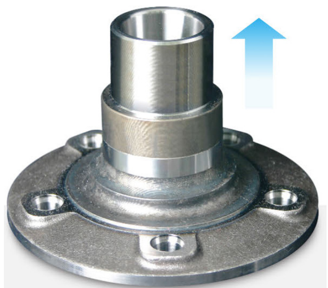
EBC16S: beschichtetes PCBN für Wälzlagerstahl: Bauteil- und Bearbeitungsansicht.
