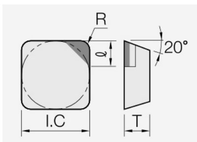
SEGN (PCD / CVD): Schneidplattenmaßzeichnung mit den zugehörigen Geometriezeichen.
