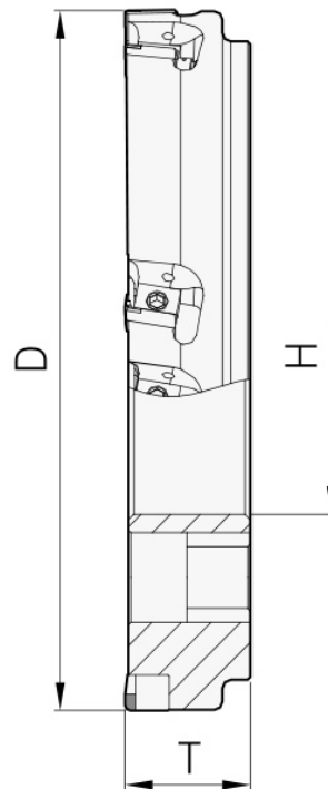
Stahl-Fräskörper und PCBN-Platten: Werkzeugansicht.
