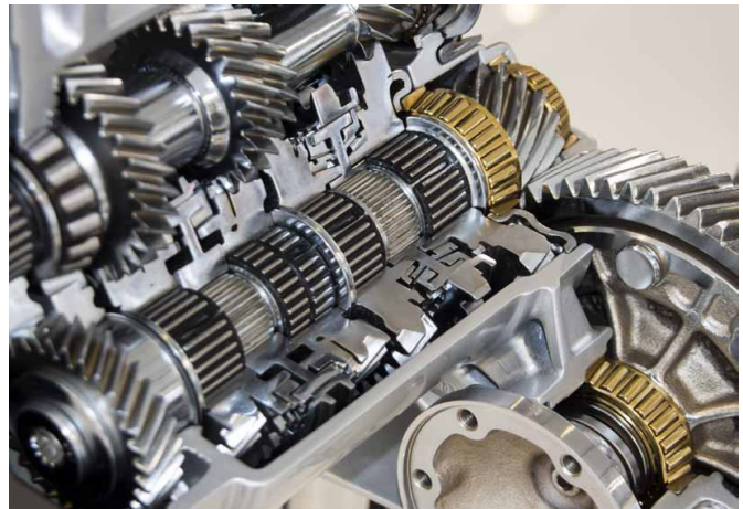
Getriebewellen: Bauteil- und Bearbeitungsansicht.
