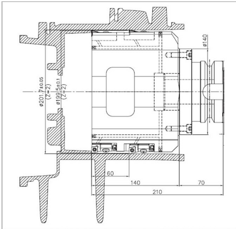
Motorgehäuse: vollständige Maßzeichnung.
