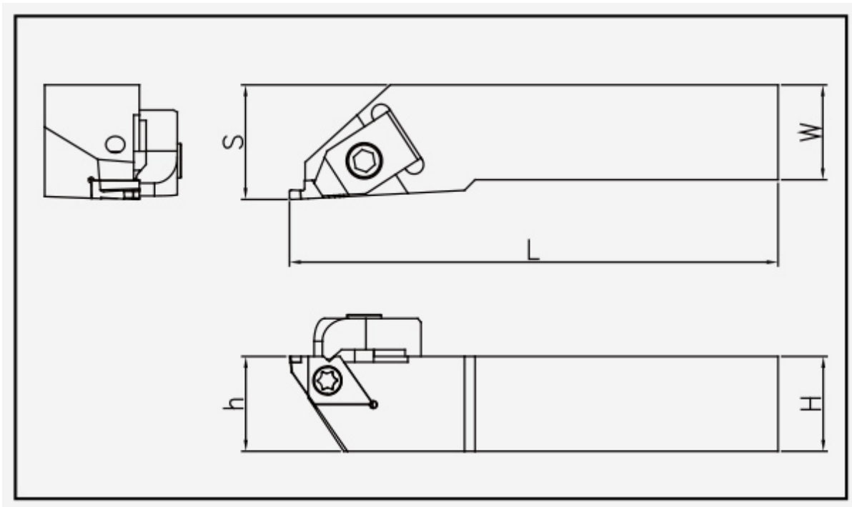
EDEH: Haltermaßzeichnung; Artikelmaße und Ersatzteile stehen in den zugehörigen Tabellen.
