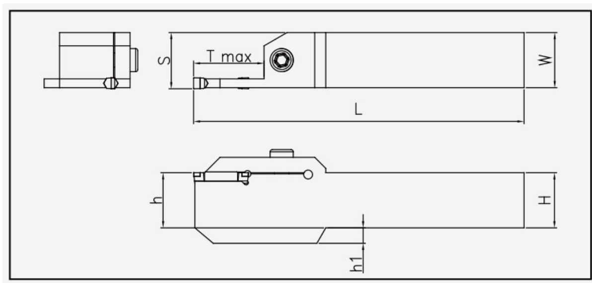
ESEH: Haltermaßzeichnung; Artikelmaße und Ersatzteile stehen in den zugehörigen Tabellen.
