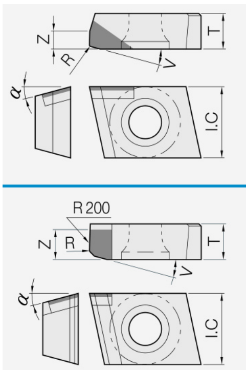
Schneidplatte: isoliertes Maßbild mit unveränderten Geometriezeichen.
