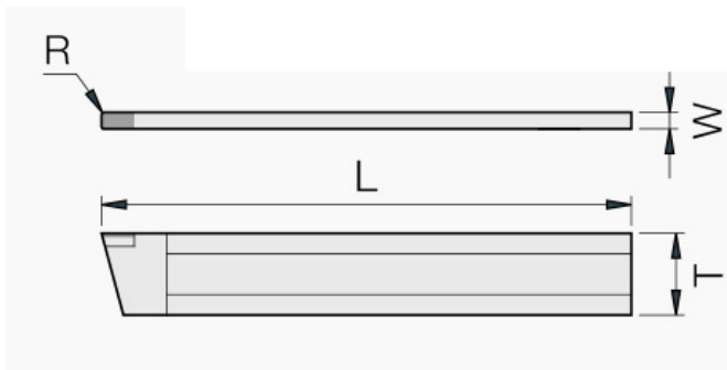
Sonderform: beide ursprünglichen Werkzeugansichten mit ihren Maßbezügen.
