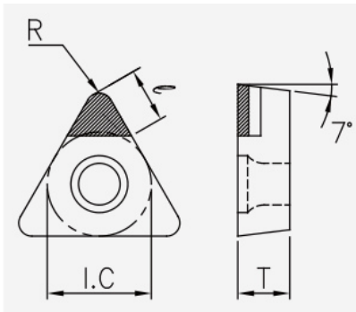
TCGW (PCD / CVD): Schneidplattenmaßzeichnung mit den zugehörigen Geometriezeichen.
