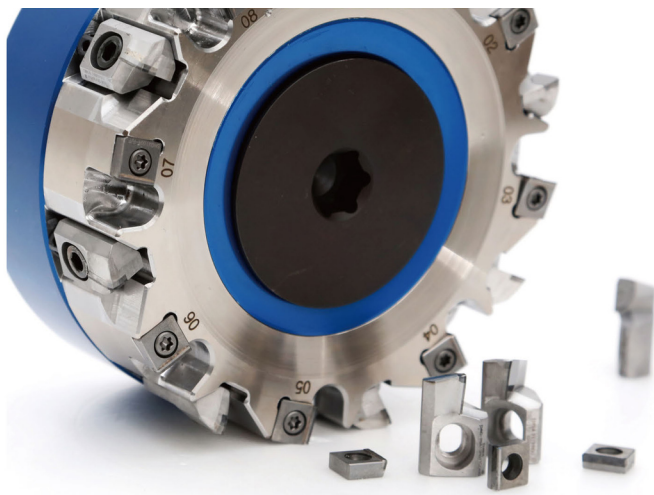
XF-Planfräser für Aluminiumlegierungen: Werkzeugansicht.
