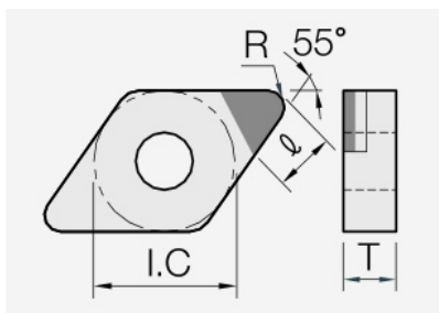
DNGA (PCBN): Schneidplattenmaßzeichnung mit den zugehörigen Geometriezeichen.
