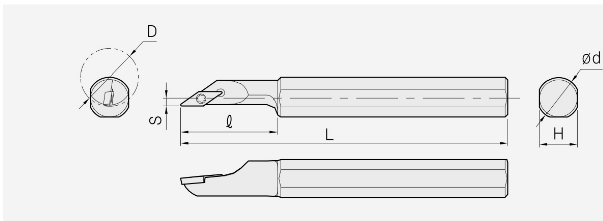
SVJC: Haltermaßzeichnung; Artikelmaße und Ersatzteile stehen in den zugehörigen Tabellen.
