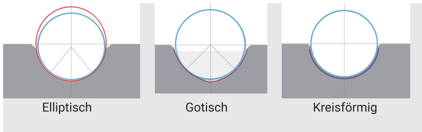
Elliptische, gotische und kreisförmige Kugelbahnprofile.
