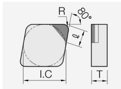
CNGN (PCBN): Schneidplattenmaßzeichnung mit den zugehörigen Geometriezeichen.
