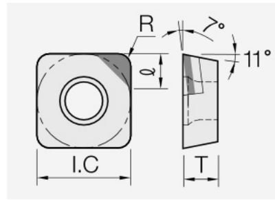
SPGT (PCD / CVD): Schneidplattenmaßzeichnung mit den zugehörigen Geometriezeichen.
