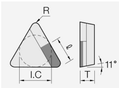
TPGN (R) (PCD / CVD): Schneidplattenmaßzeichnung mit den zugehörigen Geometriezeichen.
