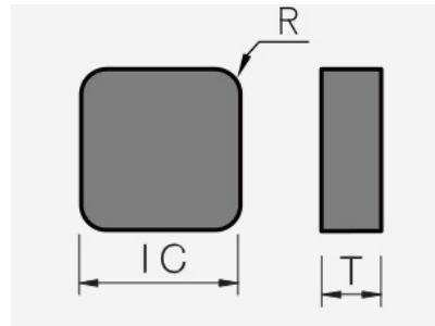
SNGN (solid) (PCBN): Schneidplattenmaßzeichnung mit den zugehörigen Geometriezeichen.
