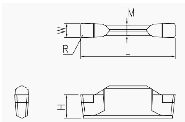
Schneidplatte: isoliertes Maßbild mit unveränderten Geometriezeichen.
