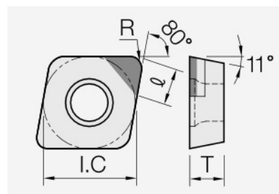
CPGW (PCBN): Schneidplattenmaßzeichnung mit den zugehörigen Geometriezeichen.
