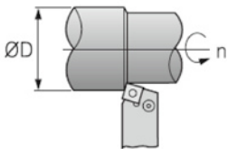
Drehen: Durchmesser D und Drehzahl N im Schnittgeschwindigkeitsmodell.
