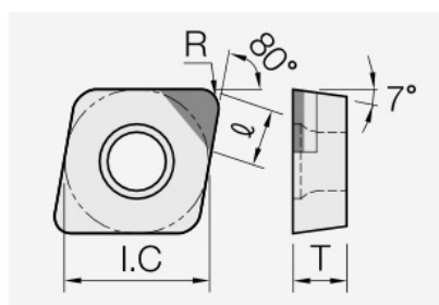
CCGW (PCD / CVD): Schneidplattenmaßzeichnung mit den zugehörigen Geometriezeichen.
