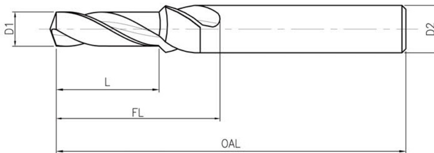
Spiralbohrer: geometrische Maßzuordnung.
