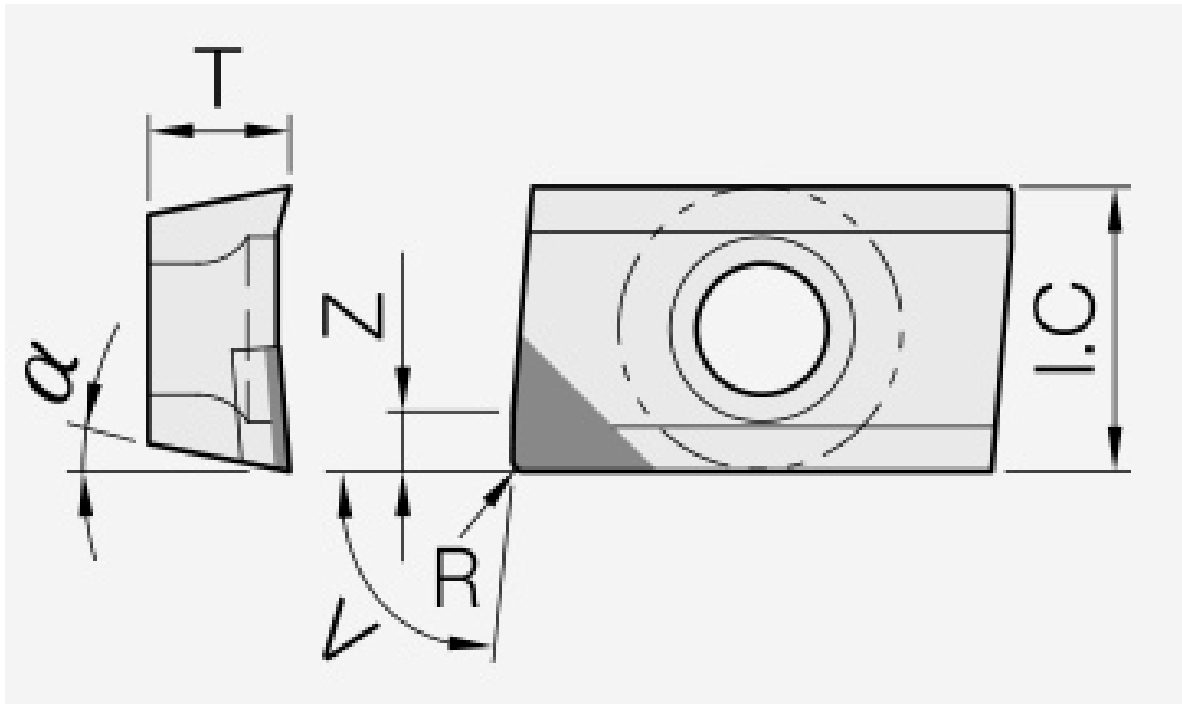
Schneidplatte: isoliertes Maßbild mit unveränderten Geometriezeichen.
