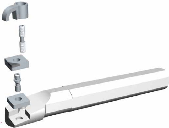
Innenhalter: Doppel- und Mehrfachspannung: Werkzeugansicht.
