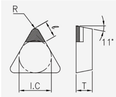
TPGN (PCD / CVD): Schneidplattenmaßzeichnung mit den zugehörigen Geometriezeichen.
