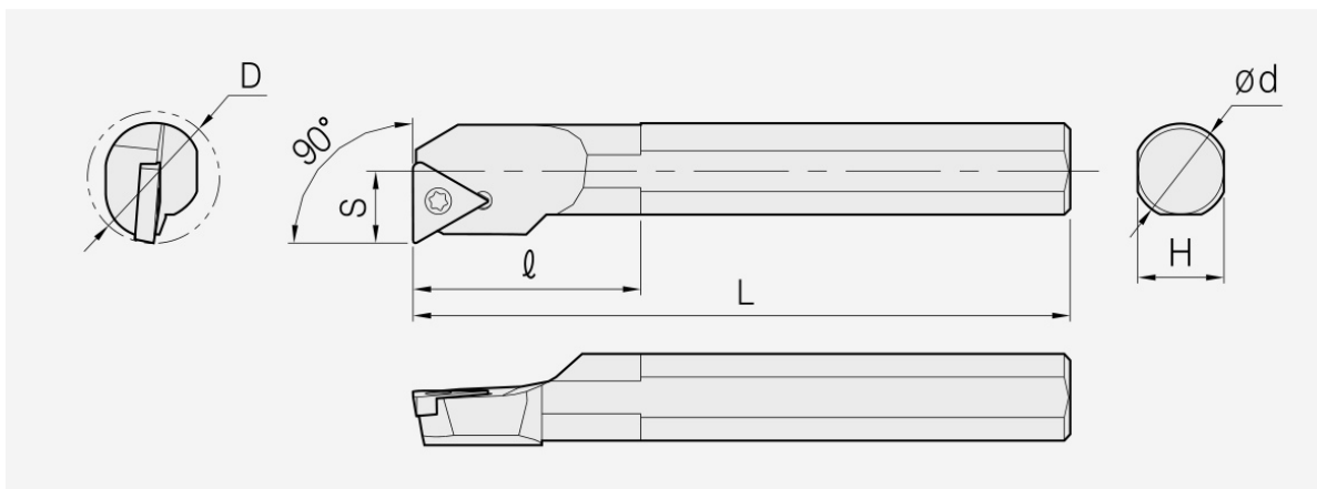
STFC: Haltermaßzeichnung; Artikelmaße und Ersatzteile stehen in den zugehörigen Tabellen.
