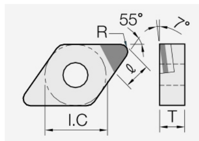
DNGX (PCD / CVD): Schneidplattenmaßzeichnung mit den zugehörigen Geometriezeichen.
