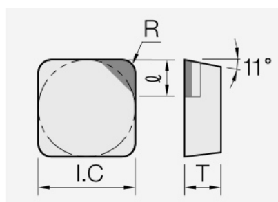
SPGN (PCBN): Schneidplattenmaßzeichnung mit den zugehörigen Geometriezeichen.
