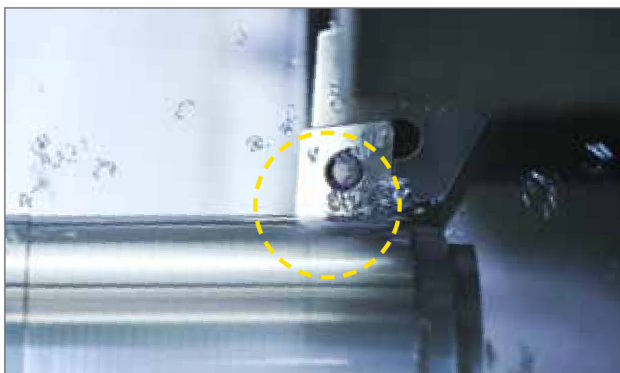
PCBN-Spanbrecher: SCM420-Anwendungsbeispiele: Bauteil- und Bearbeitungsansicht.
