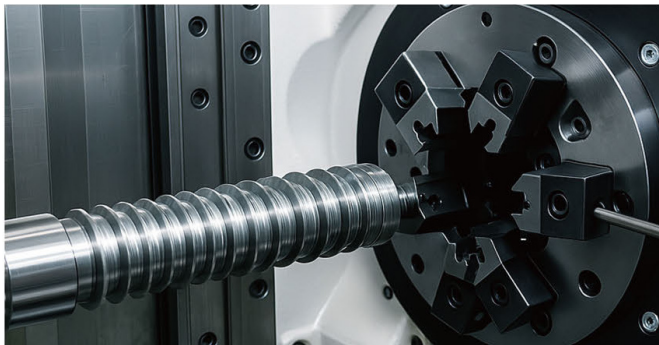
Gewindewirbeln: Geometrie, Sorten und Beschichtungen: Bauteil- und Bearbeitungsansicht.
