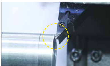
PKD-Spanbrecher: Aluminium-Anwendungsbeispiele: Bauteil- und Bearbeitungsansicht.
