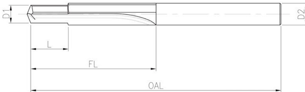
Glättbohrer: Maßschema D1, D2, L, FL und OAL.
