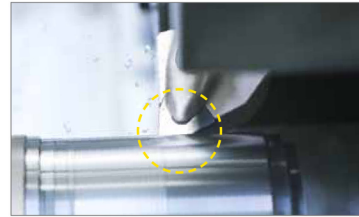
PCBN-Spanbrecher: SCM420-Anwendungsbeispiele: Bauteil- und Bearbeitungsansicht.
