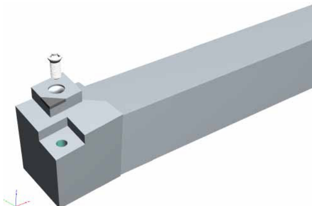
Mehrfach- und Schraubenspannung: Aufbau: Werkzeugansicht.
