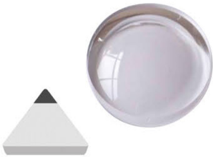
PKD-Sorten EP20, EP55 und EP59: Bauteil- und Bearbeitungsansicht.
