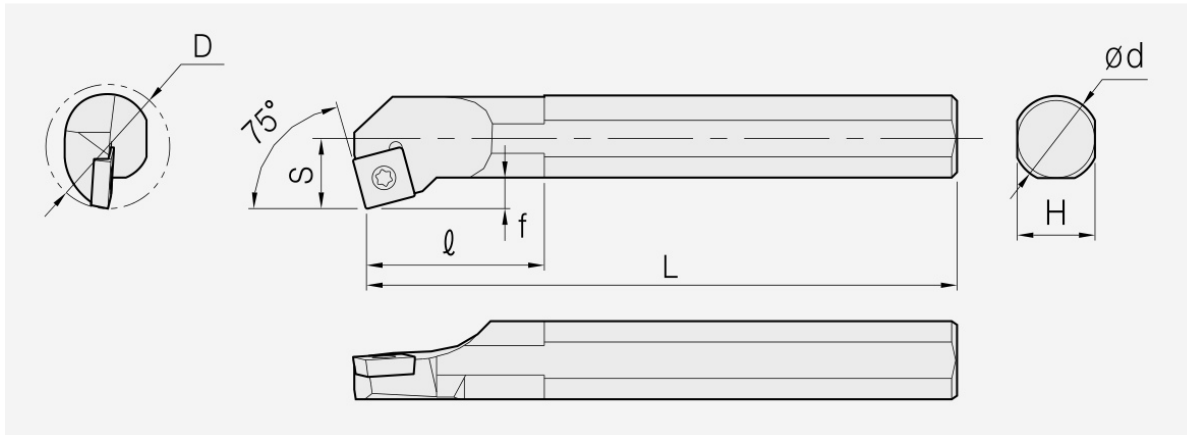
SSKP: Haltermaßzeichnung; Artikelmaße und Ersatzteile stehen in den zugehörigen Tabellen.
