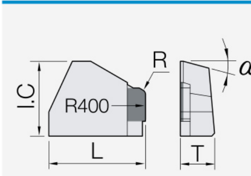
Schneidplatte: isoliertes Maßbild mit unveränderten Geometriezeichen.
