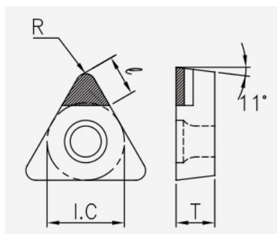
TPGW (PCBN): Schneidplattenmaßzeichnung mit den zugehörigen Geometriezeichen.
