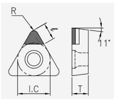
TPGW (PCD / CVD): Schneidplattenmaßzeichnung mit den zugehörigen Geometriezeichen.
