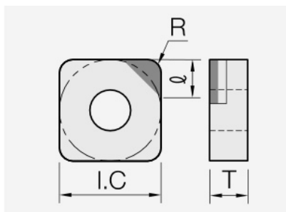
SNGA (PCD / CVD): Schneidplattenmaßzeichnung mit den zugehörigen Geometriezeichen.
