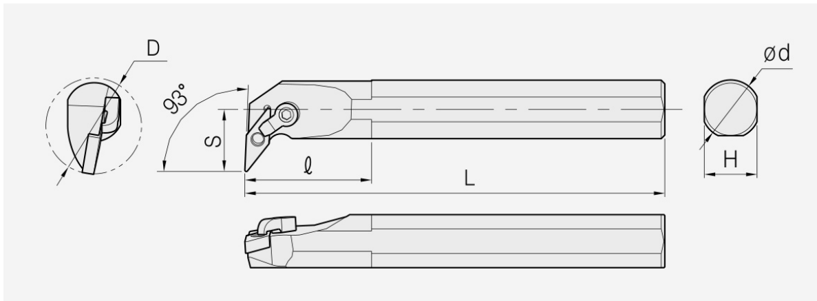
MVUN: Haltermaßzeichnung; Artikelmaße und Ersatzteile stehen in den zugehörigen Tabellen.
