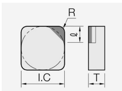
SNGN (PCD / CVD): Schneidplattenmaßzeichnung mit den zugehörigen Geometriezeichen.
