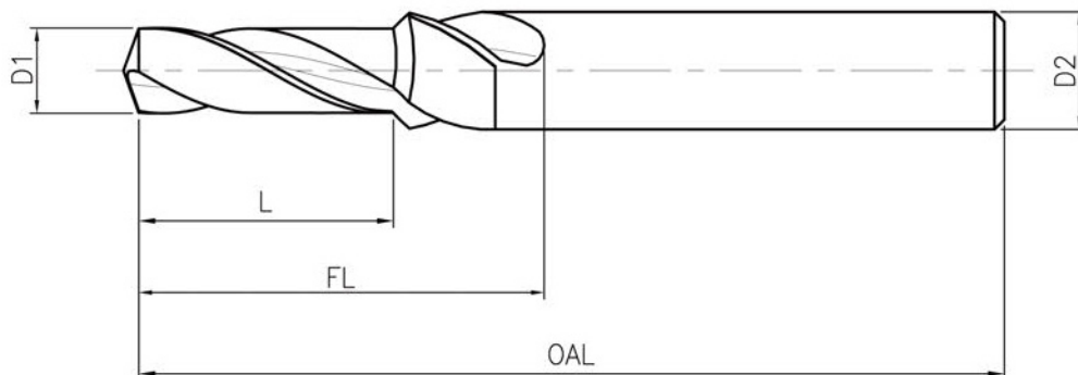
Spiralbohrer: Maßschema D1, D2, L, FL und OAL.
