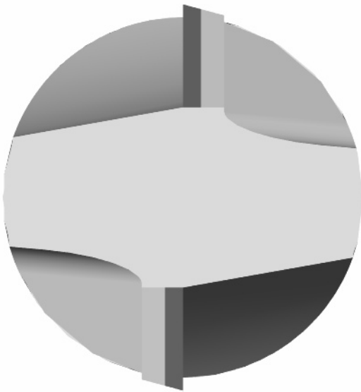
PKD-Reibahlen: Standard und Spanbrecher: Werkzeugansicht.
