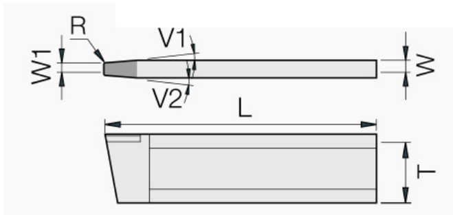
Sonderform: beide ursprünglichen Werkzeugansichten mit ihren Maßbezügen.
