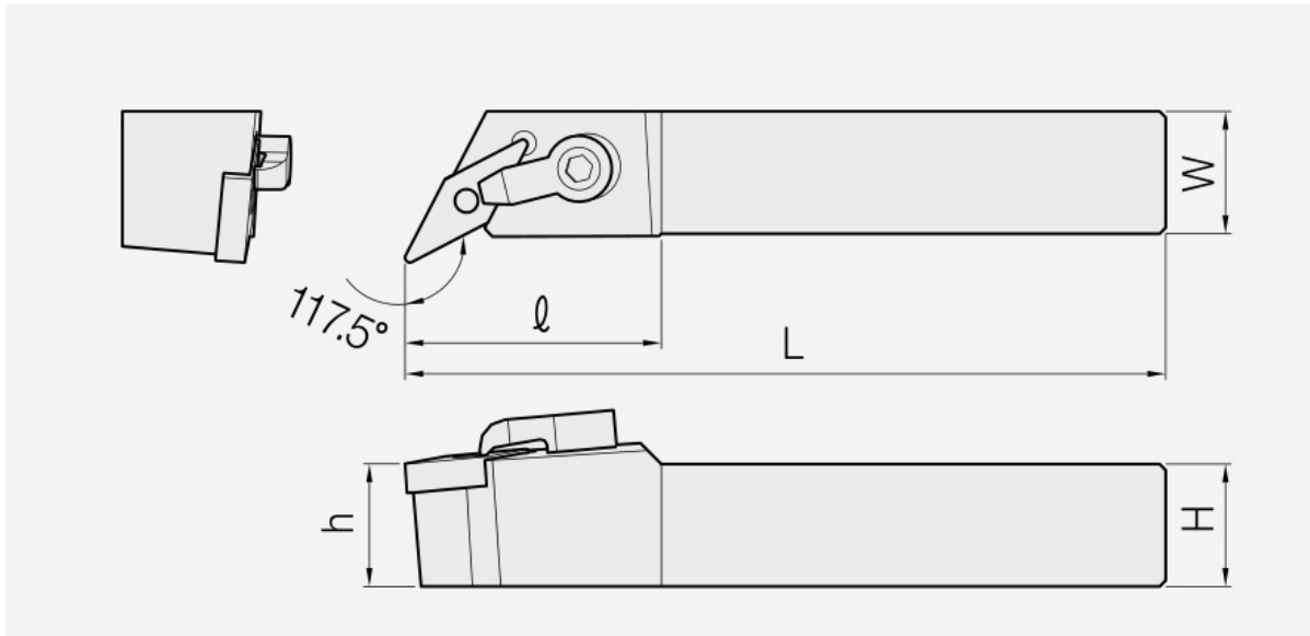
MVQN: Haltermaßzeichnung; Artikelmaße und Ersatzteile stehen in den zugehörigen Tabellen.
