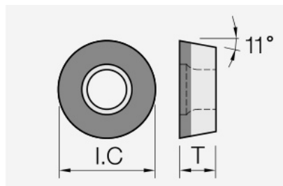
RPGW (PCD / CVD): Schneidplattenmaßzeichnung mit den zugehörigen Geometriezeichen.
