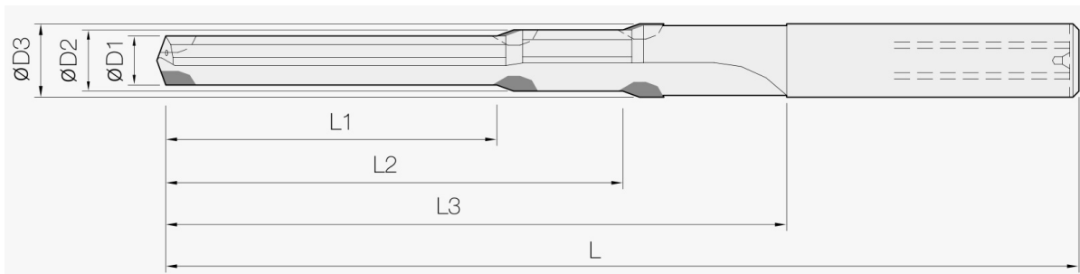
Bohrer: L1, L2 und L3 vom gemeinsamen vorderen Bezug; getrennte Stufendurchmesser.
