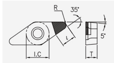
VBGW (PCBN): Schneidplattenmaßzeichnung mit den zugehörigen Geometriezeichen.
