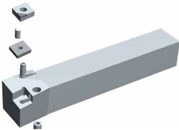
Doppel- und Hebelspannung: Aufbau: Werkzeugansicht.
