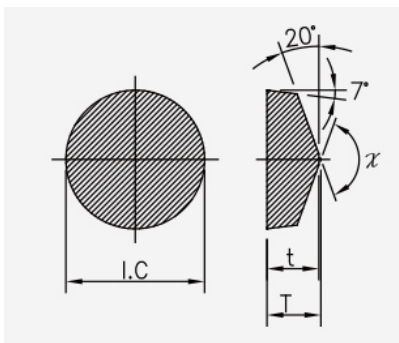
Schneidplatte: isoliertes Maßbild mit unveränderten Geometriezeichen.
