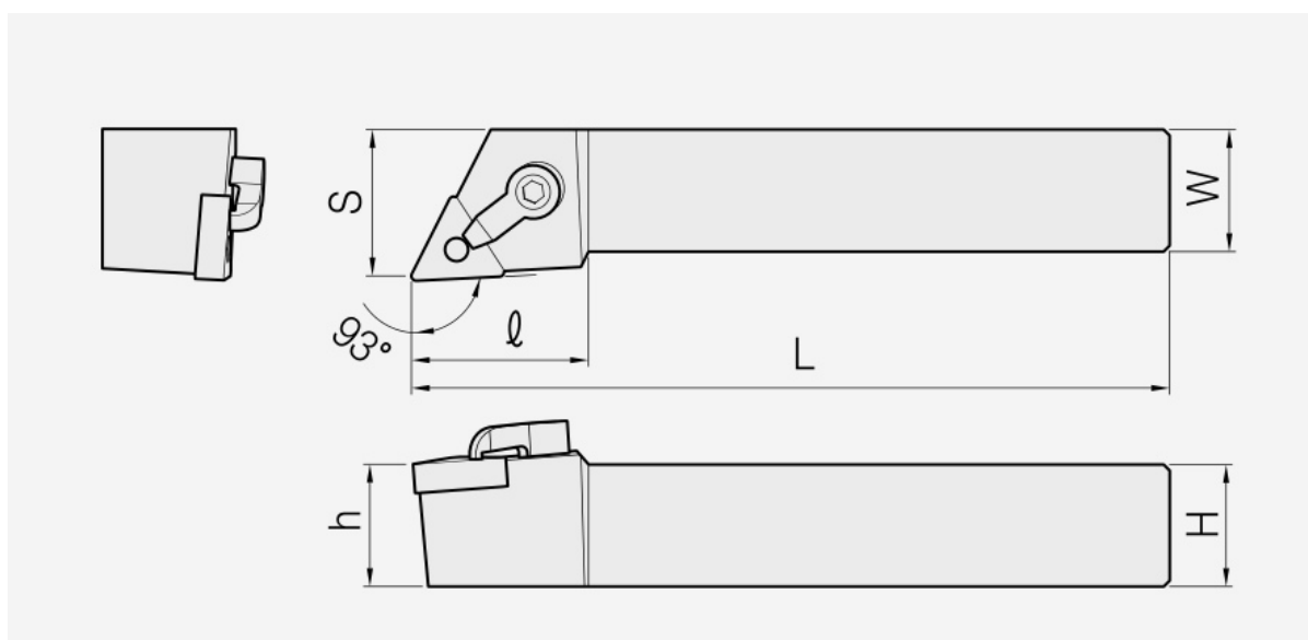
MTJN: Haltermaßzeichnung; Artikelmaße und Ersatzteile stehen in den zugehörigen Tabellen.
