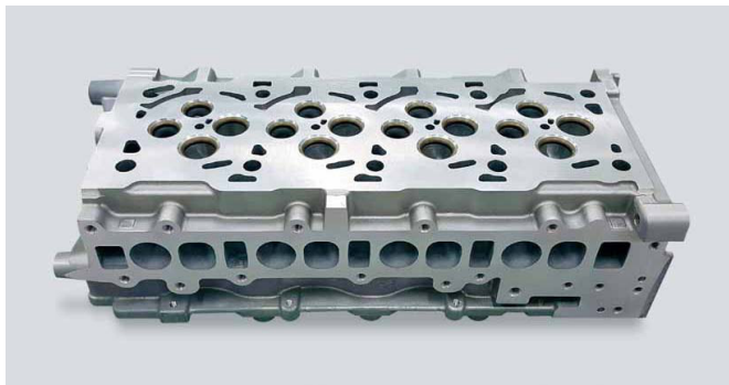
Aluminium-Zylinderkopf: Ventil- und Planflächen: Bauteil- und Bearbeitungsansicht.
