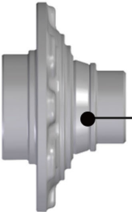
Wälzlager: Innenbearbeitung und Bohren: Bauteil- und Bearbeitungsansicht.
