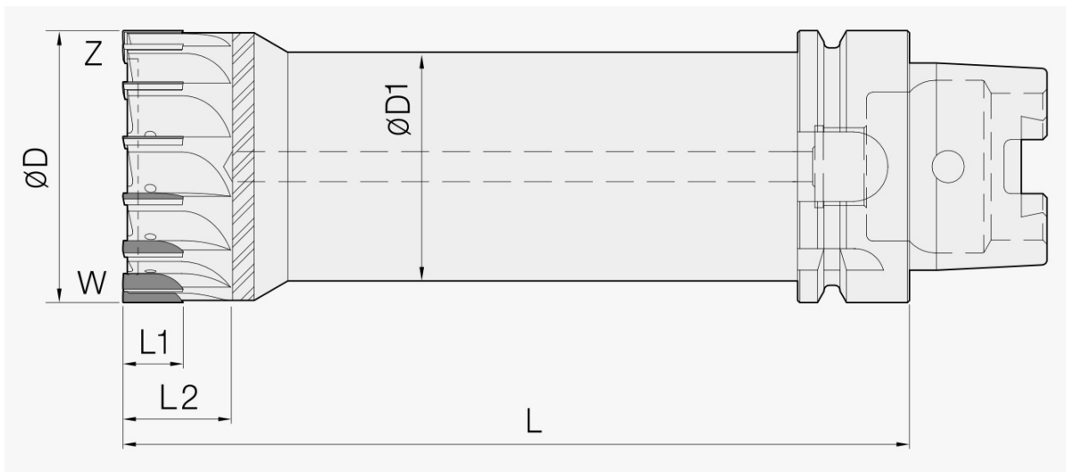
Schaftfräser: unveränderte Maßbezüge D, D1, L1, L2, W, L und Z des Auslegungsblatts.
