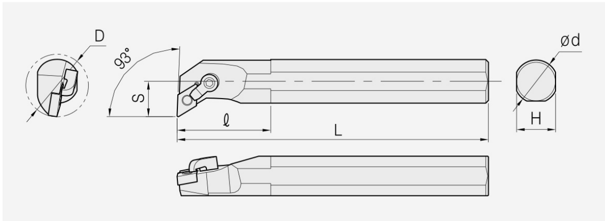
MDUN: Haltermaßzeichnung; Artikelmaße und Ersatzteile stehen in den zugehörigen Tabellen.
