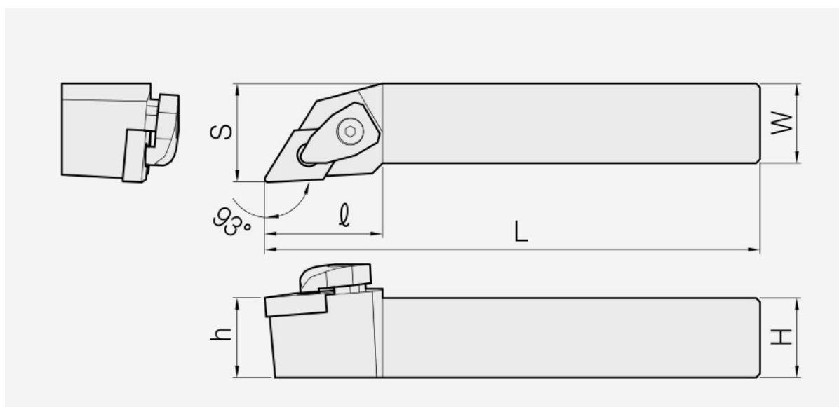
DDJN: Haltermaßzeichnung; Artikelmaße und Ersatzteile stehen in den zugehörigen Tabellen.
