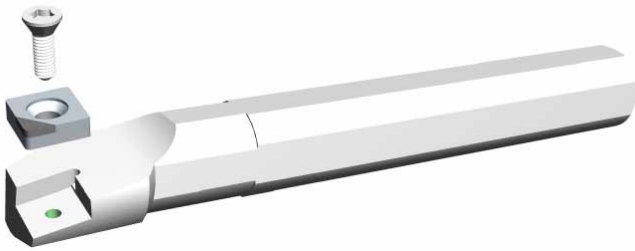
Innenhalter: Hebel- und Schraubenspannung: Werkzeugansicht.
