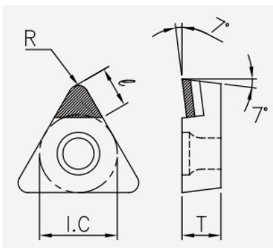
TCGT (PCD / CVD): Schneidplattenmaßzeichnung mit den zugehörigen Geometriezeichen.
