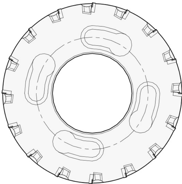
Stahl-Fräskörper und PCBN-Platten: Werkzeugansicht.
