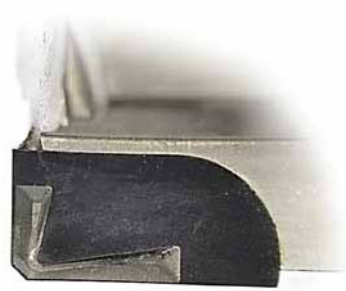
PKD-Reibahlen: Standard und Spanbrecher: Werkzeugansicht.
