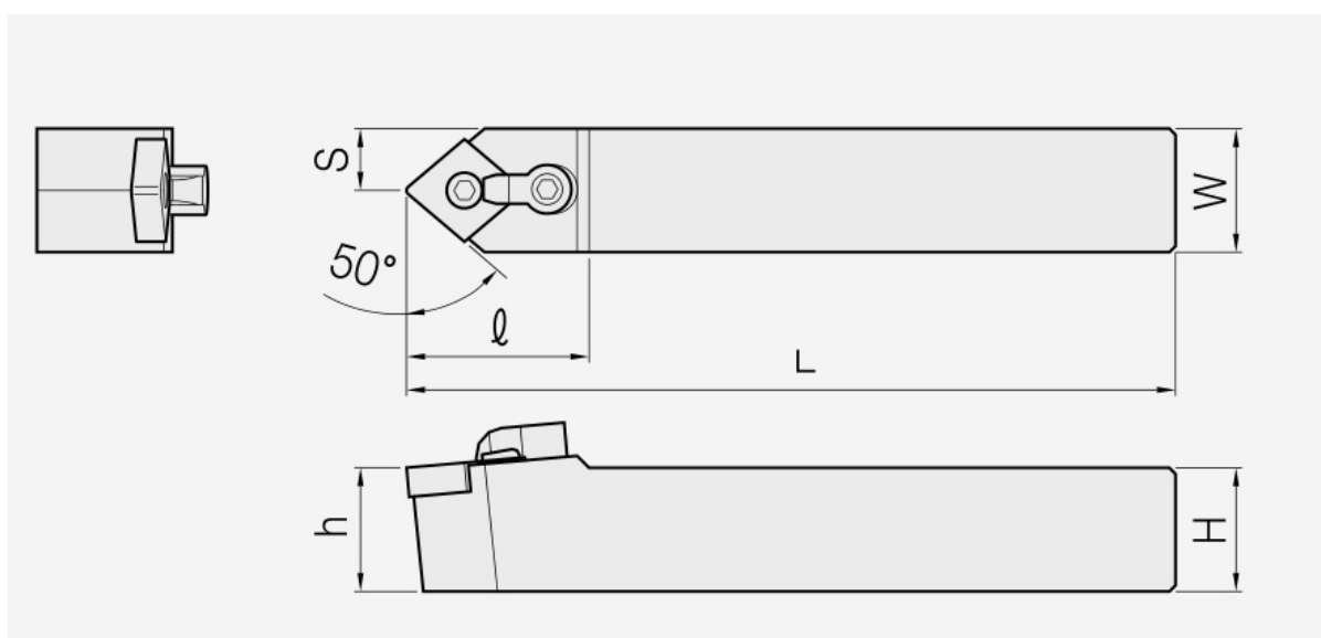
MCMNN: Haltermaßzeichnung; Artikelmaße und Ersatzteile stehen in den zugehörigen Tabellen.
