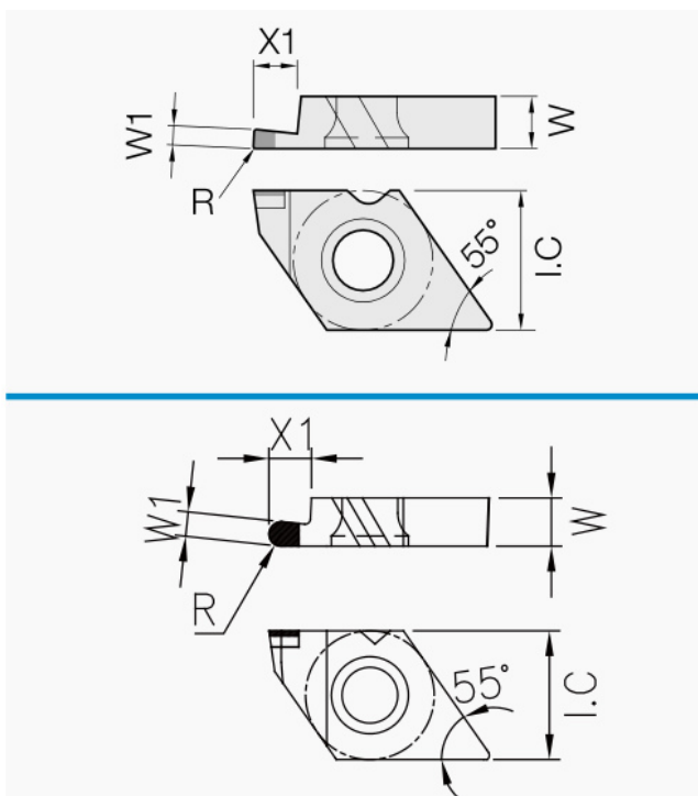
Schneidplatte: isoliertes Maßbild mit unveränderten Geometriezeichen.
