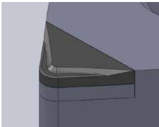
PCBN-Spanbrecher ER, EF und ES: Werkzeugansicht.
