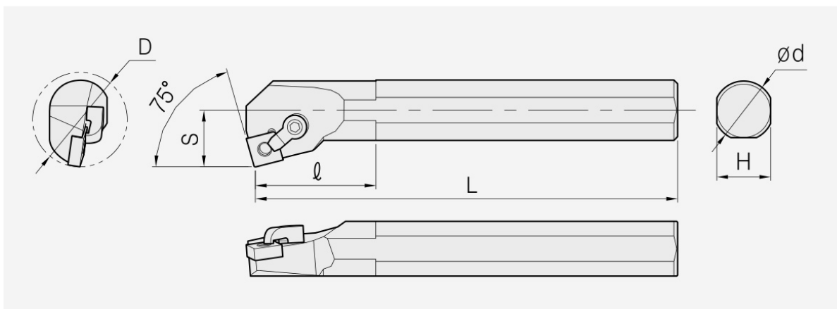
MSKN: Haltermaßzeichnung; Artikelmaße und Ersatzteile stehen in den zugehörigen Tabellen.
