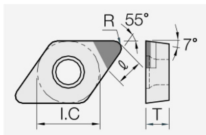
DCGW (PCBN): Schneidplattenmaßzeichnung mit den zugehörigen Geometriezeichen.
