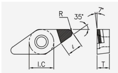
VNGX (PCD / CVD): Schneidplattenmaßzeichnung mit den zugehörigen Geometriezeichen.
