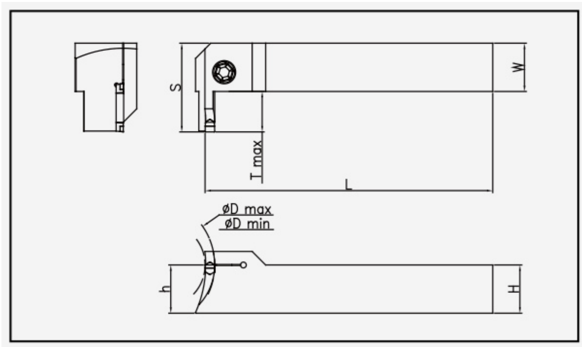
ESFV: Haltermaßzeichnung; Artikelmaße und Ersatzteile stehen in den zugehörigen Tabellen.
