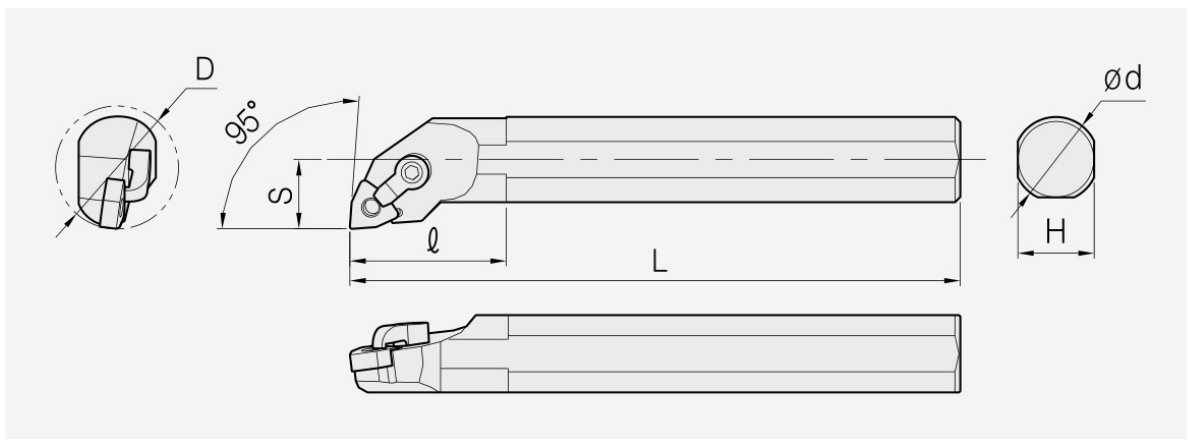
MWLN: Haltermaßzeichnung; Artikelmaße und Ersatzteile stehen in den zugehörigen Tabellen.
