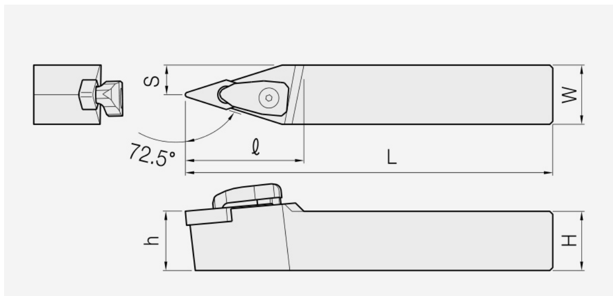
DVWNN: Haltermaßzeichnung; Artikelmaße und Ersatzteile stehen in den zugehörigen Tabellen.
