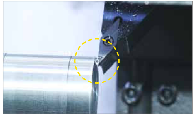
PKD-Spanbrecher: Aluminium-Anwendungsbeispiele: Bauteil- und Bearbeitungsansicht.
