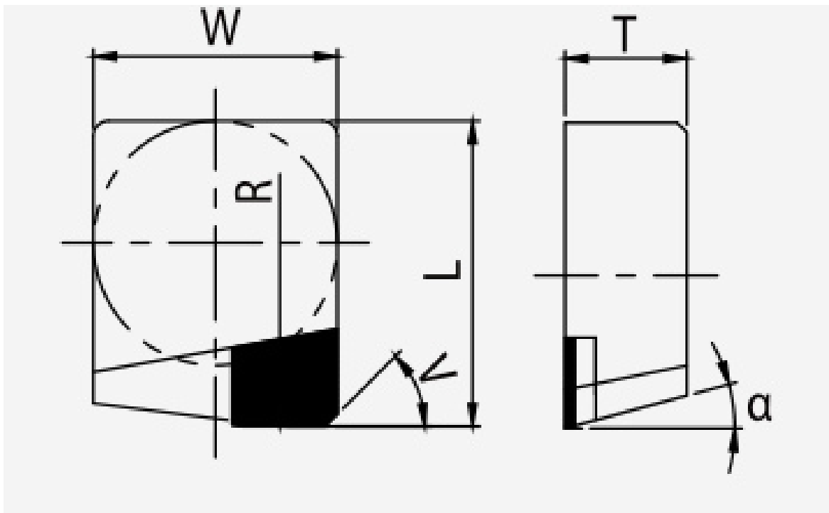
Werkzeug: isoliertes Maßbild; Ansichten und Maßbezüge unverändert.
