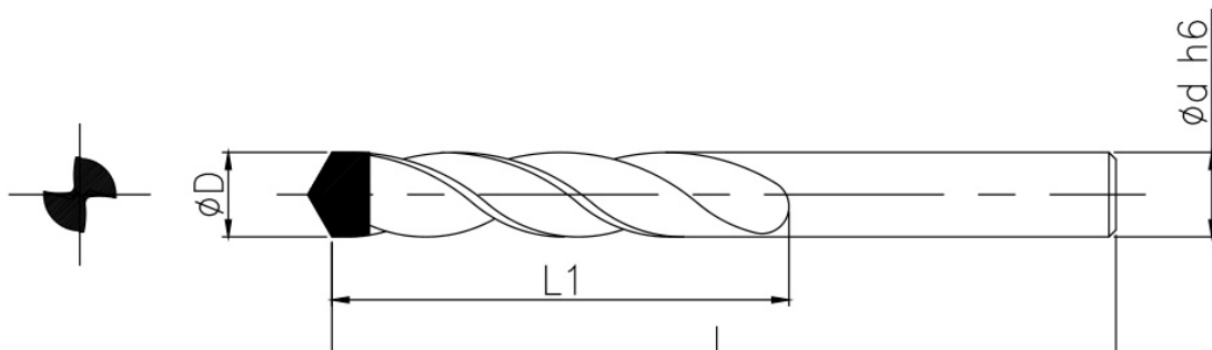
Werkzeug: isoliertes Maßbild; Ansichten und Maßbezüge unverändert.
