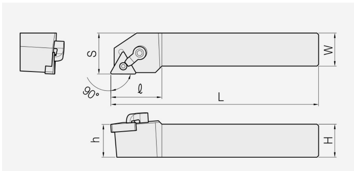
MTGN: Haltermaßzeichnung; Artikelmaße und Ersatzteile stehen in den zugehörigen Tabellen.
