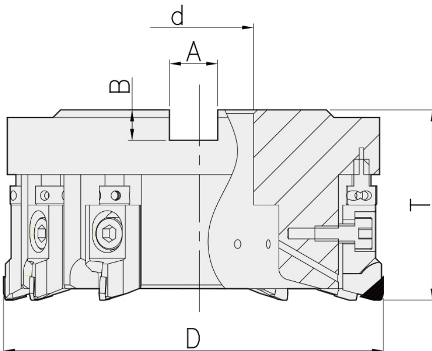
Werkzeug: isoliertes Maßbild; Ansichten und Maßbezüge unverändert.
