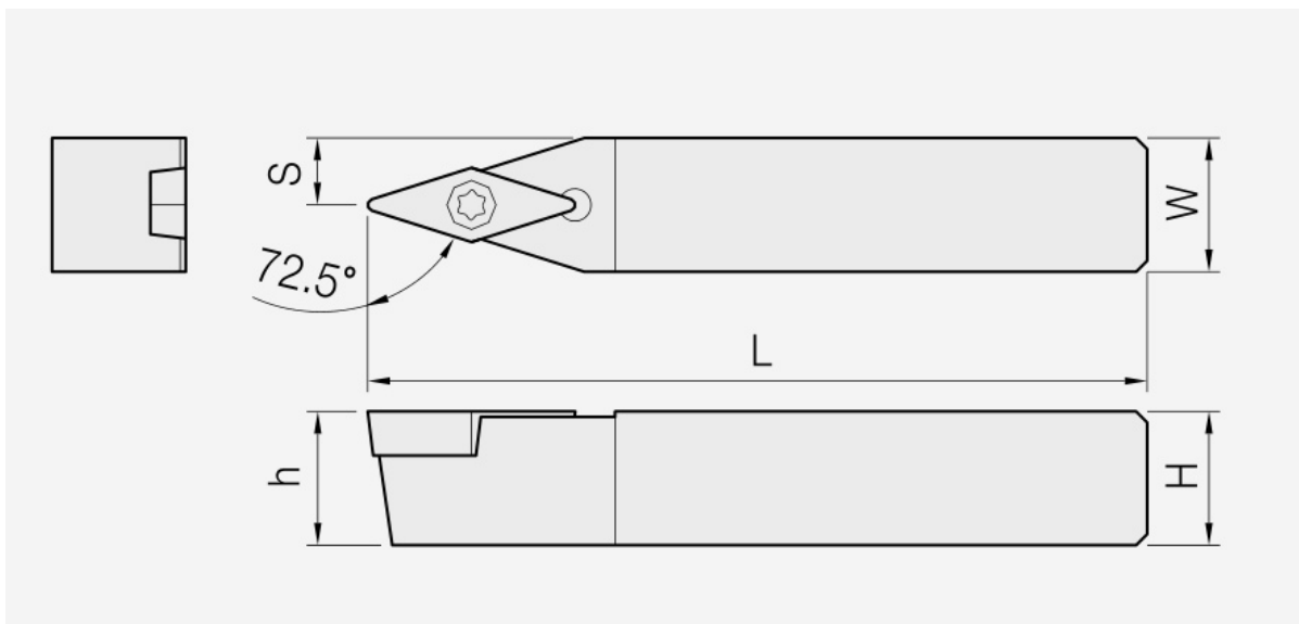
SVBVB: Haltermaßzeichnung; Artikelmaße und Ersatzteile stehen in den zugehörigen Tabellen.
