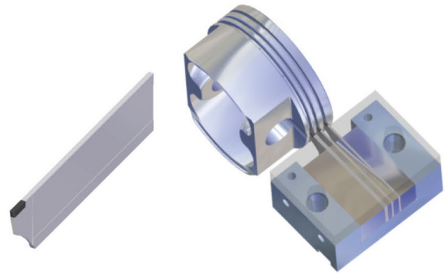
Nut- und Abstechwerkzeuge, Gewindewirbeln und Kolben: Bauteil- und Bearbeitungsansicht.
