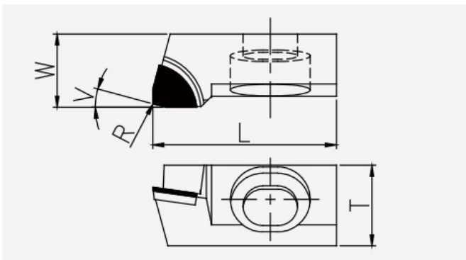
Schneidplatte: isoliertes Maßbild mit unveränderten Geometriezeichen.
