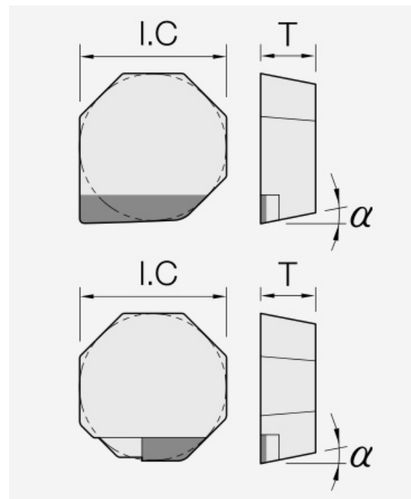
Schneidplatte: isoliertes Maßbild mit unveränderten Geometriezeichen.
