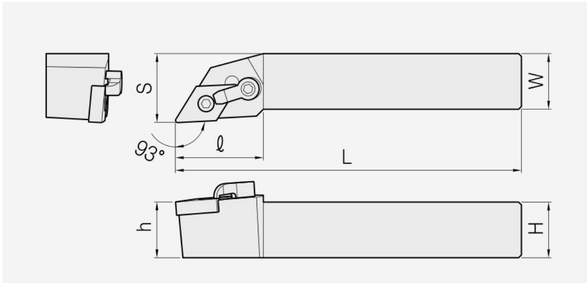
MDJN: Haltermaßzeichnung; Artikelmaße und Ersatzteile stehen in den zugehörigen Tabellen.
