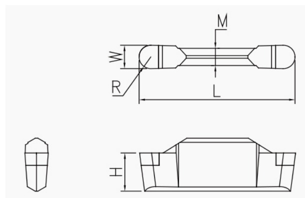
Schneidplatte: isoliertes Maßbild mit unveränderten Geometriezeichen.
