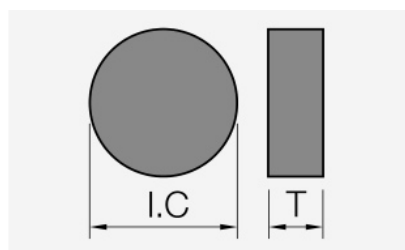
RNGN (solid) (PCBN): Schneidplattenmaßzeichnung mit den zugehörigen Geometriezeichen.
