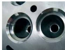
Aluminium-Zylinderkopf: Ventil- und Planflächen: Bauteil- und Bearbeitungsansicht.
