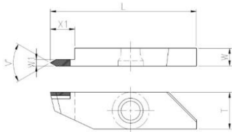
EMT: Zeichnung mit W1, X1, T, W, L und V.
