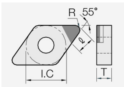
DNGA (PCD / CVD): Schneidplattenmaßzeichnung mit den zugehörigen Geometriezeichen.
