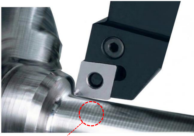
Illustrative Bearbeitungsansicht ohne Wiper.
