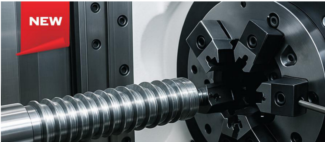
Gewindewirbeln eines Spindelbauteils.
