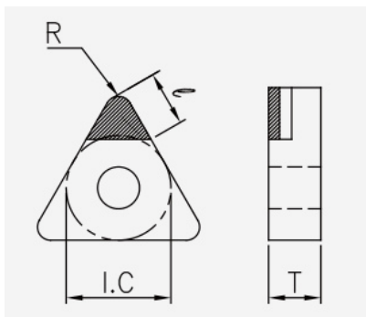
TNGA (PCD / CVD): Schneidplattenmaßzeichnung mit den zugehörigen Geometriezeichen.
