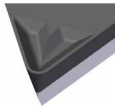
PKD-/CVD-Spanbrecher EF und ES: Werkzeugansicht.
