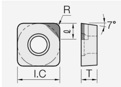
SCGW (PCD / CVD): Schneidplattenmaßzeichnung mit den zugehörigen Geometriezeichen.
