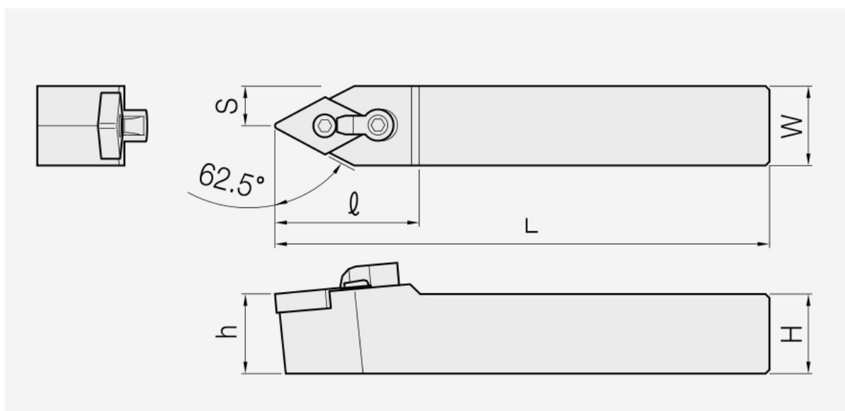
MDNNN: Haltermaßzeichnung; Artikelmaße und Ersatzteile stehen in den zugehörigen Tabellen.
