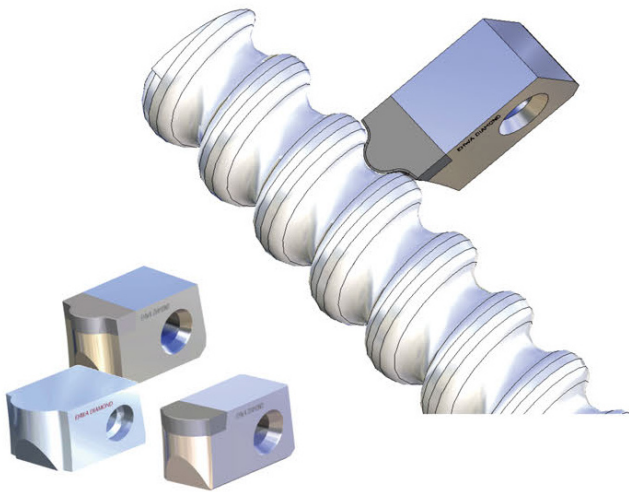
Nut- und Abstechwerkzeuge, Gewindewirbeln und Kolben: Werkzeugsansicht.
