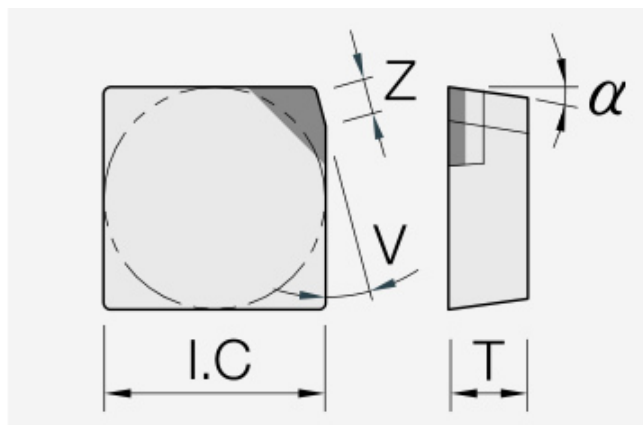
Schneidplatte: isoliertes Maßbild mit unveränderten Geometriezeichen.
