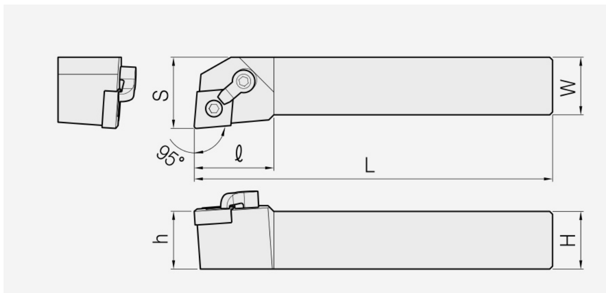
MCLN: Haltermaßzeichnung; Artikelmaße und Ersatzteile stehen in den zugehörigen Tabellen.
