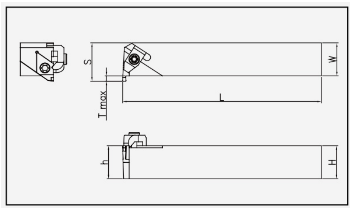
EDEV: Haltermaßzeichnung; Artikelmaße und Ersatzteile stehen in den zugehörigen Tabellen.
