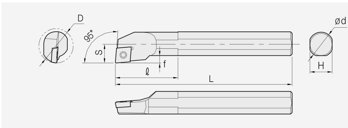
SCLP: Haltermaßzeichnung; Artikelmaße und Ersatzteile stehen in den zugehörigen Tabellen.
