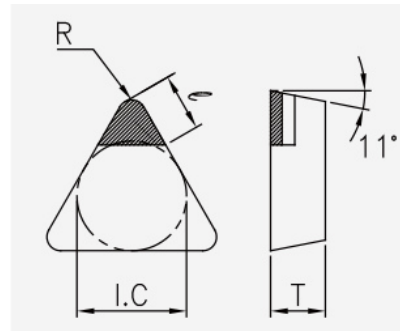
TPGN (PCBN): Schneidplattenmaßzeichnung mit den zugehörigen Geometriezeichen.
