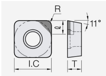
SPGW (PCD / CVD): Schneidplattenmaßzeichnung mit den zugehörigen Geometriezeichen.
