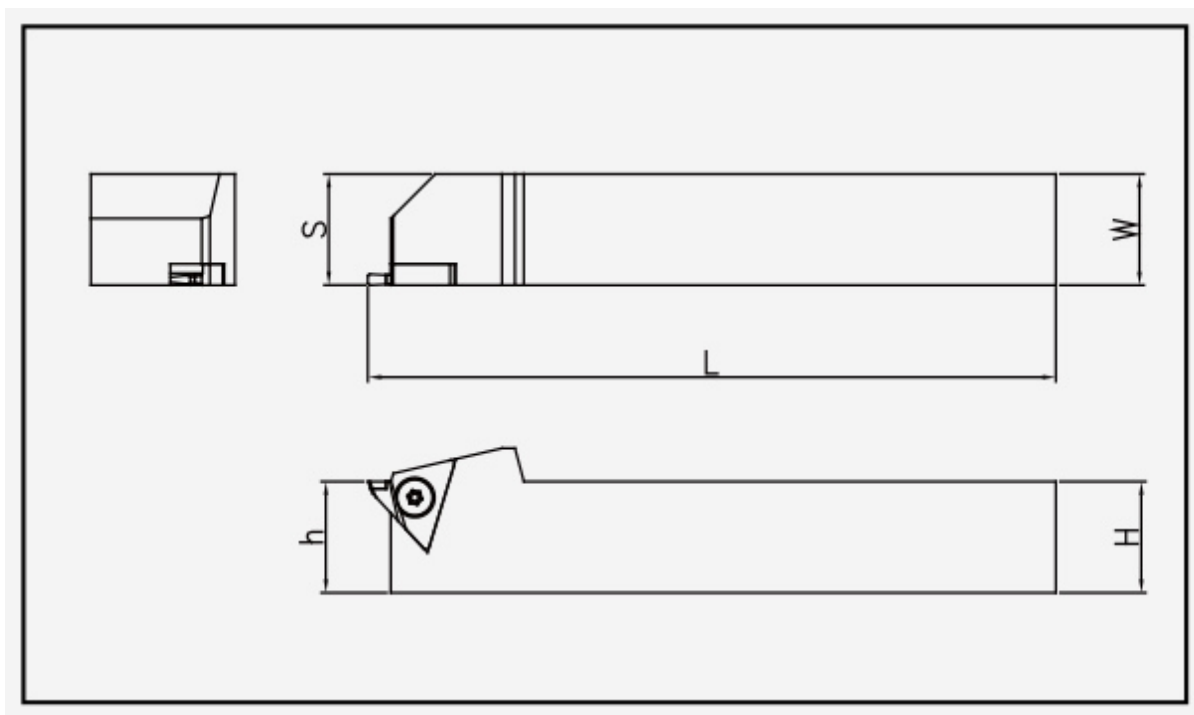
ETEH: Haltermaßzeichnung; Artikelmaße und Ersatzteile stehen in den zugehörigen Tabellen.
