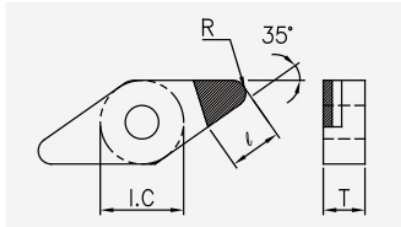
VNGA (PCBN): Schneidplattenmaßzeichnung mit den zugehörigen Geometriezeichen.
