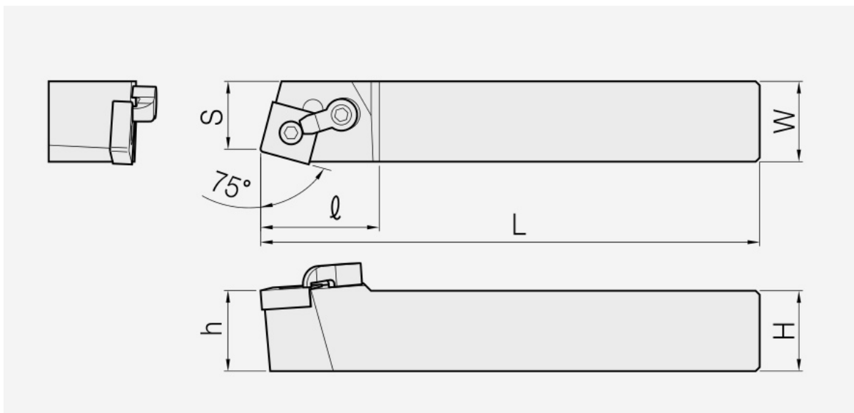
MSBN: Haltermaßzeichnung; Artikelmaße und Ersatzteile stehen in den zugehörigen Tabellen.
