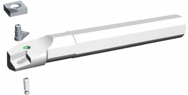
Innenhalter: Hebel- und Schraubenspannung: Werkzeugansicht.
