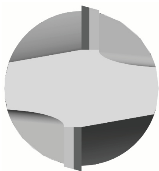
EBEB: PCBN-Kugelfräser: Werkzeugansicht.
