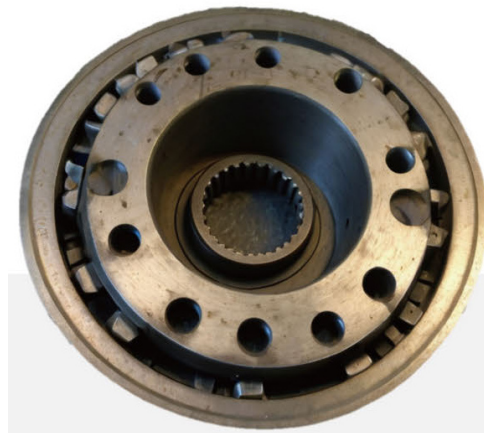
EB319: beschichtetes PCBN für gehärteten Stahl: Bauteil- und Bearbeitungsansicht.
