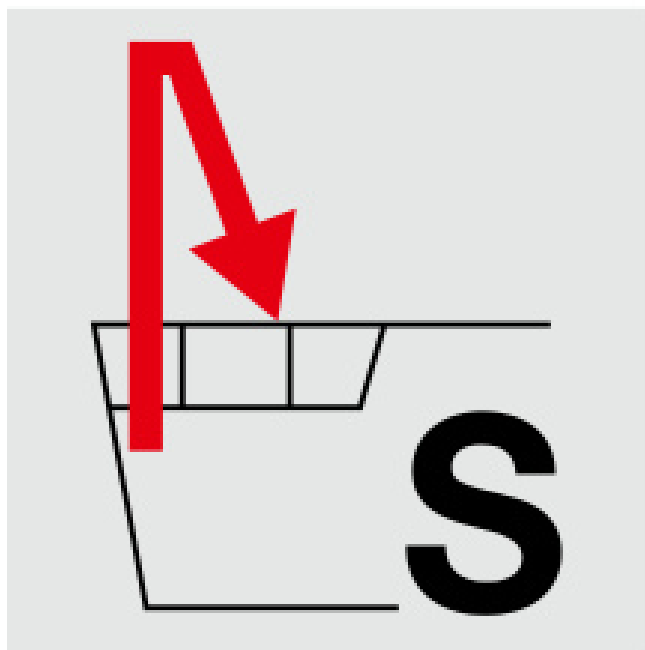
Spannsprinzip S: unveränderte Pfeilrichtungen.
