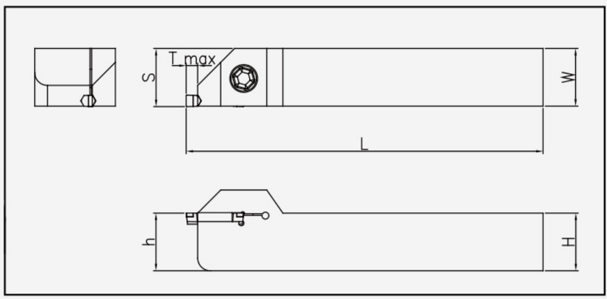
ESEH-T00: Haltermaßzeichnung; Artikelmaße und Ersatzteile stehen in den zugehörigen Tabellen.
