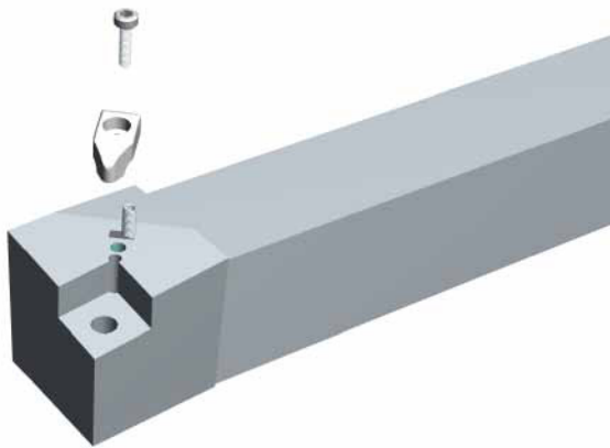
Doppel- und Hebelspannung: Aufbau: Werkzeugansicht.
