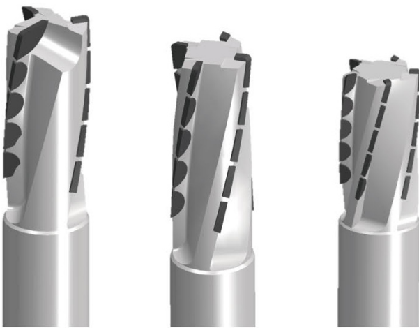
PKD-Schaftfräser für Elektrofahrzeuge: Werkzeugansicht.
