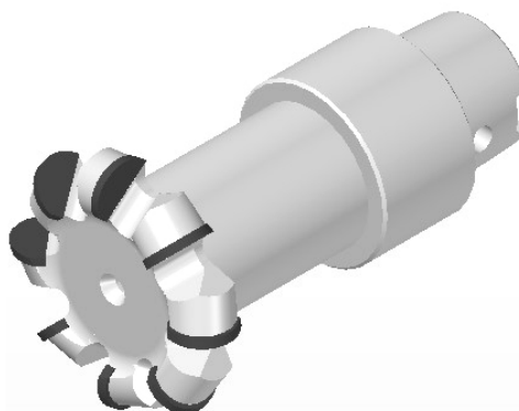
Design 45D-8Z-HSK32C.
